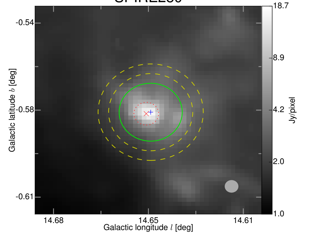
SPIRE250
