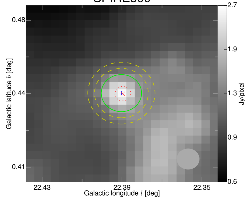
SPIRE500
