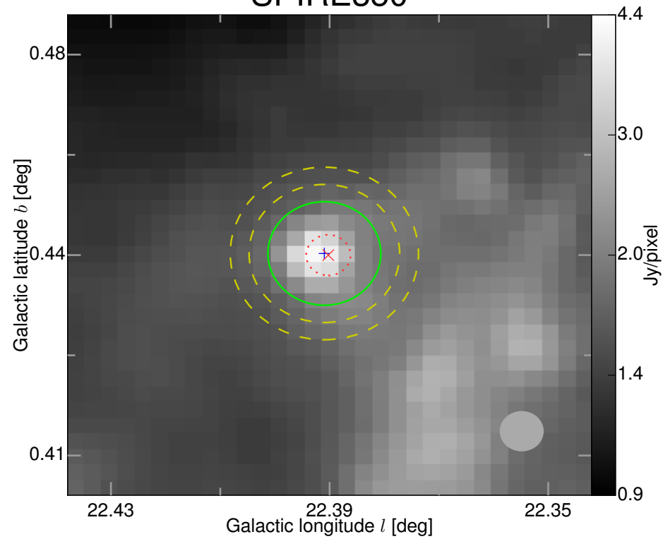
SPIRE350
