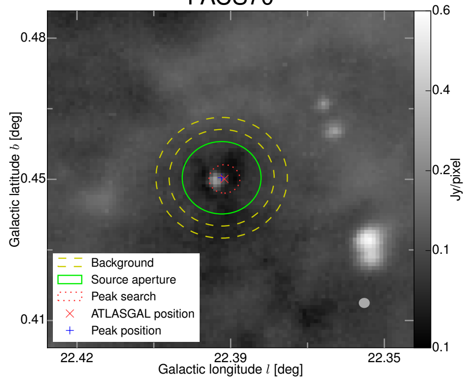
PACS70
