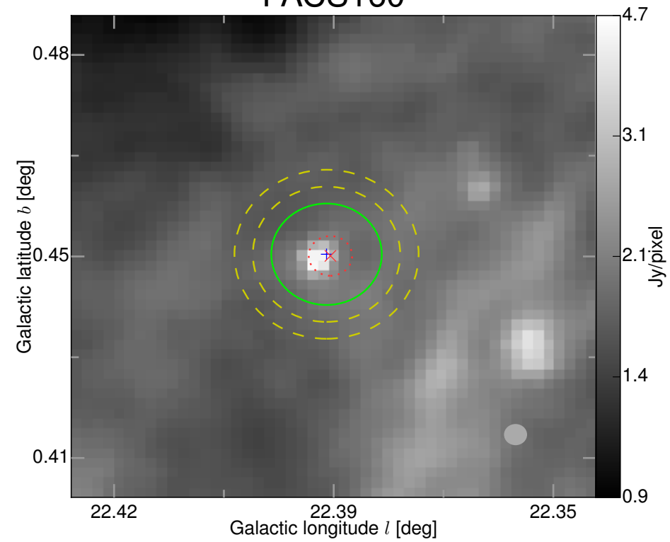
PACS160
