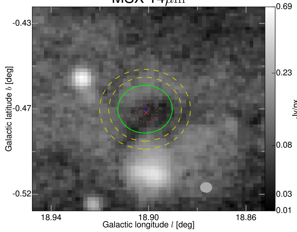
MSX 14\mu\text{m}
