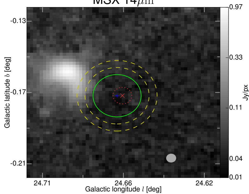
MSX 14 \mu\text{m}
