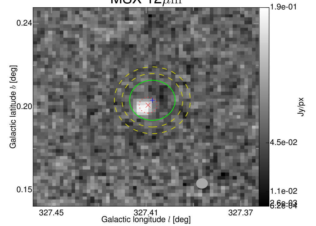
MSX 12\mu\text{m}
