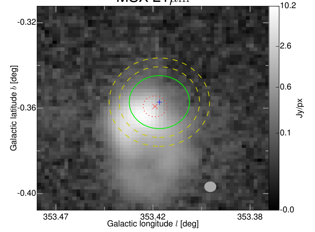
MSX 21 \mu m
