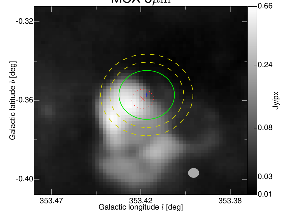
MSX 8 \mu m
