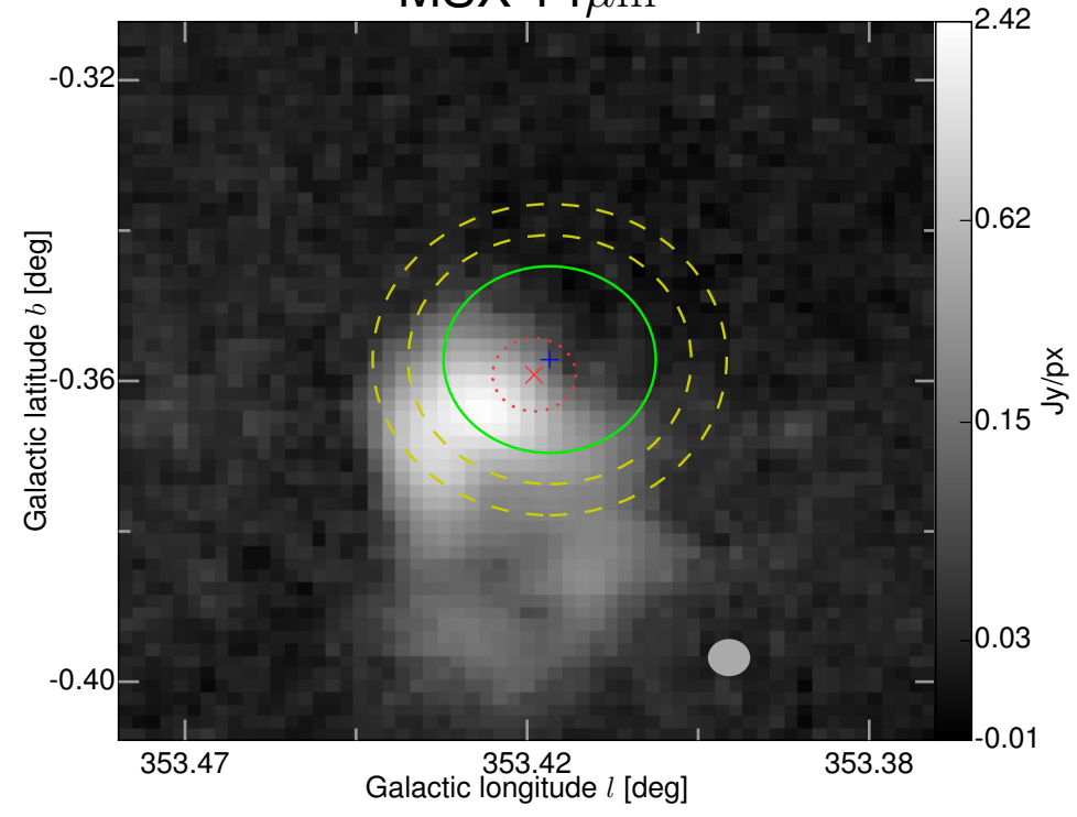
MSX 14 \mu m
