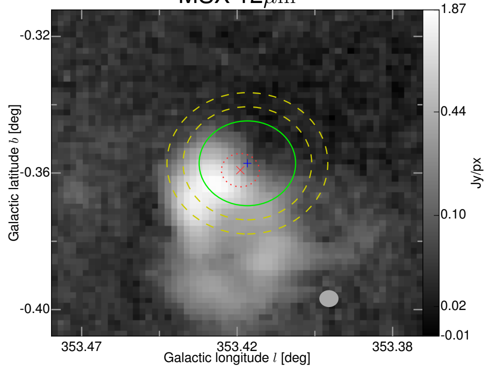
MSX 12 \mu m
