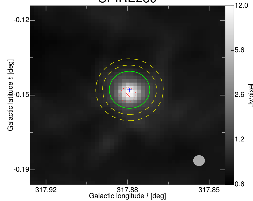
SPIRE250
