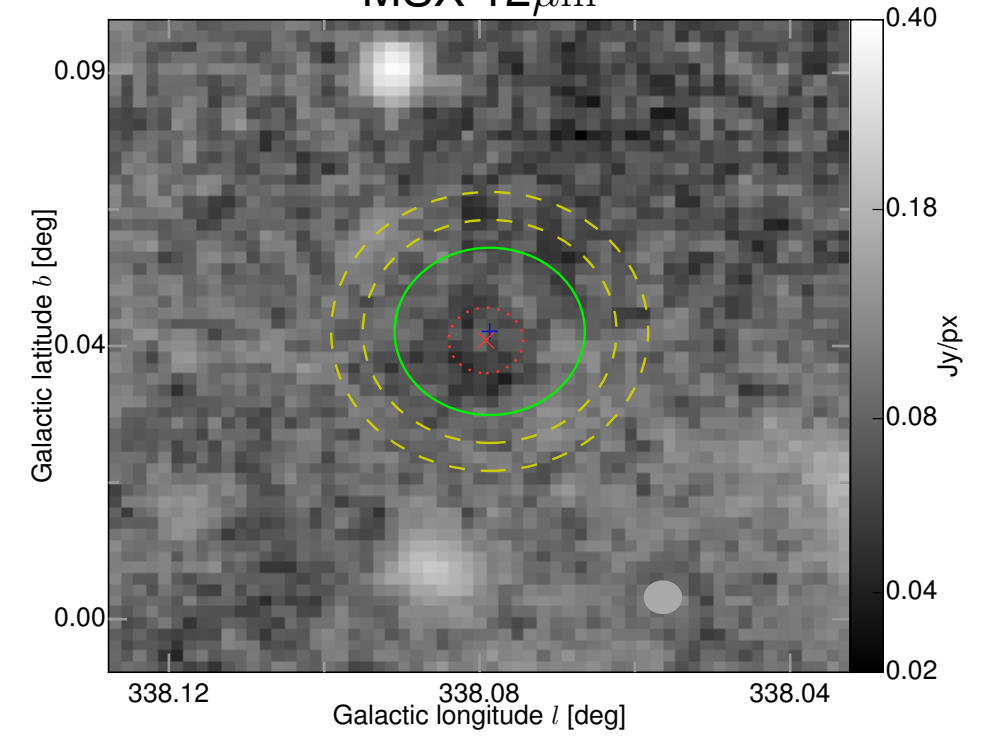
MSX 12\mu\text{m}
