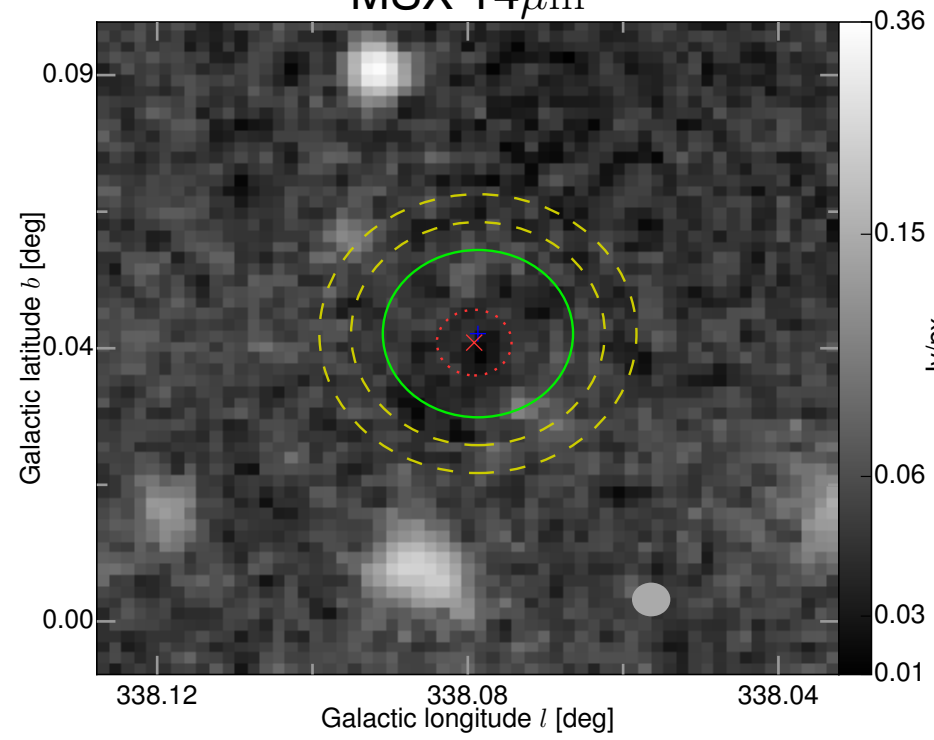
MSX 14\mu\text{m}
