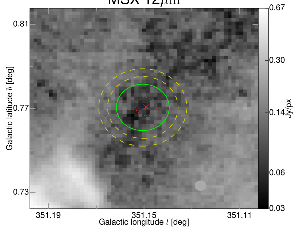
MSX 12\mu\text{m}
