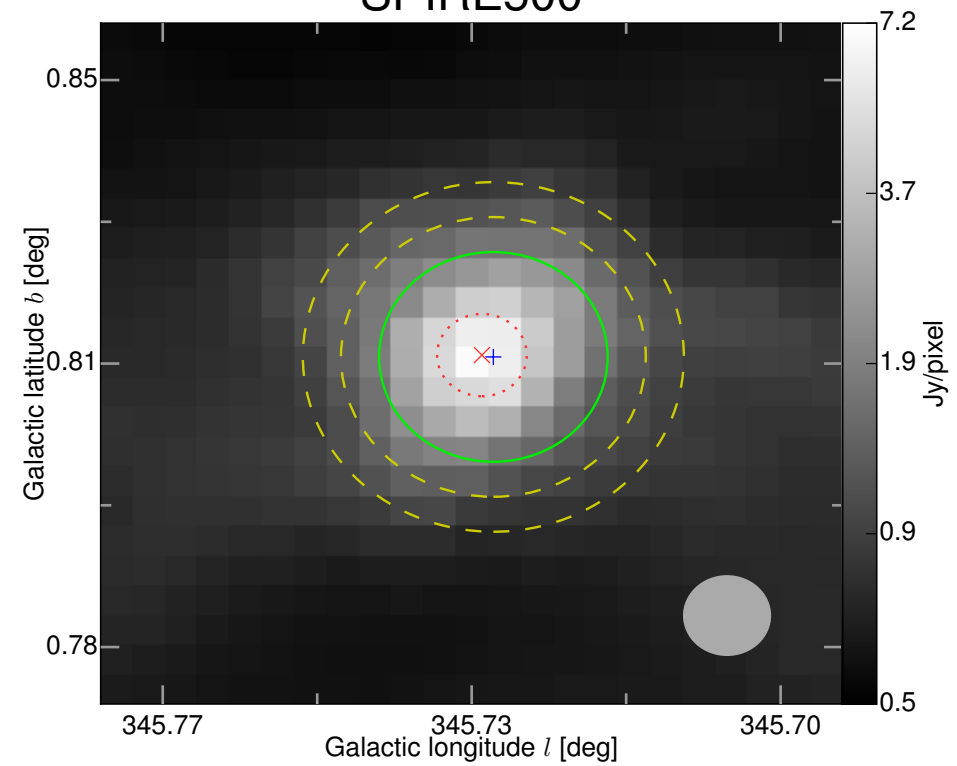
SPIRE500
