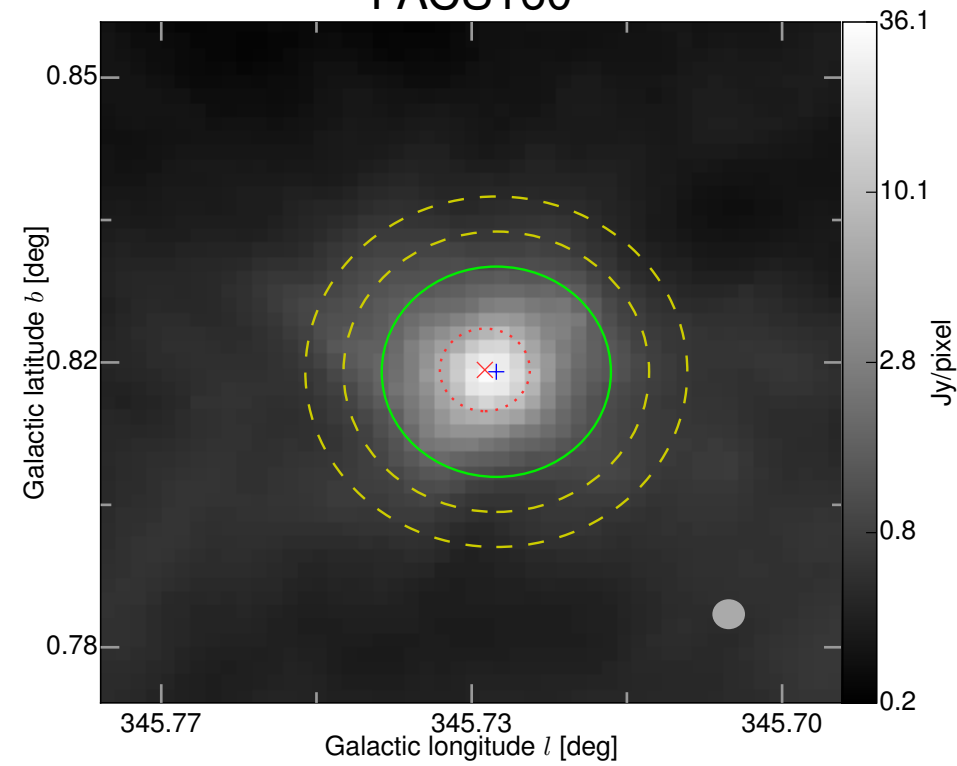
PACS160
