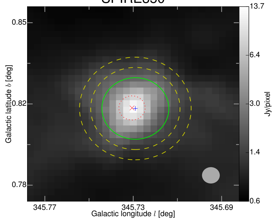
SPIRE350
