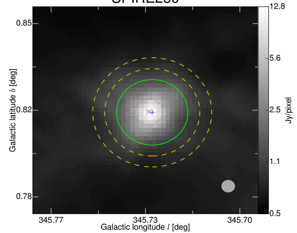
SPIRE250
