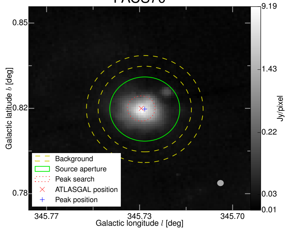
PACS70
