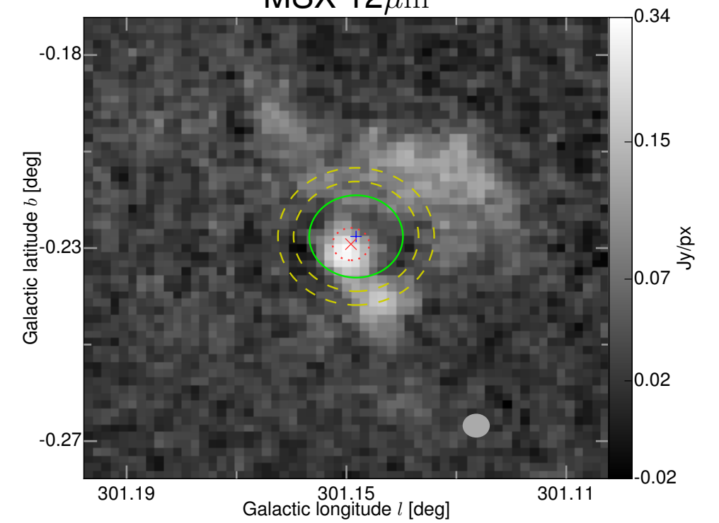
MSX 12\mu\text{m}
