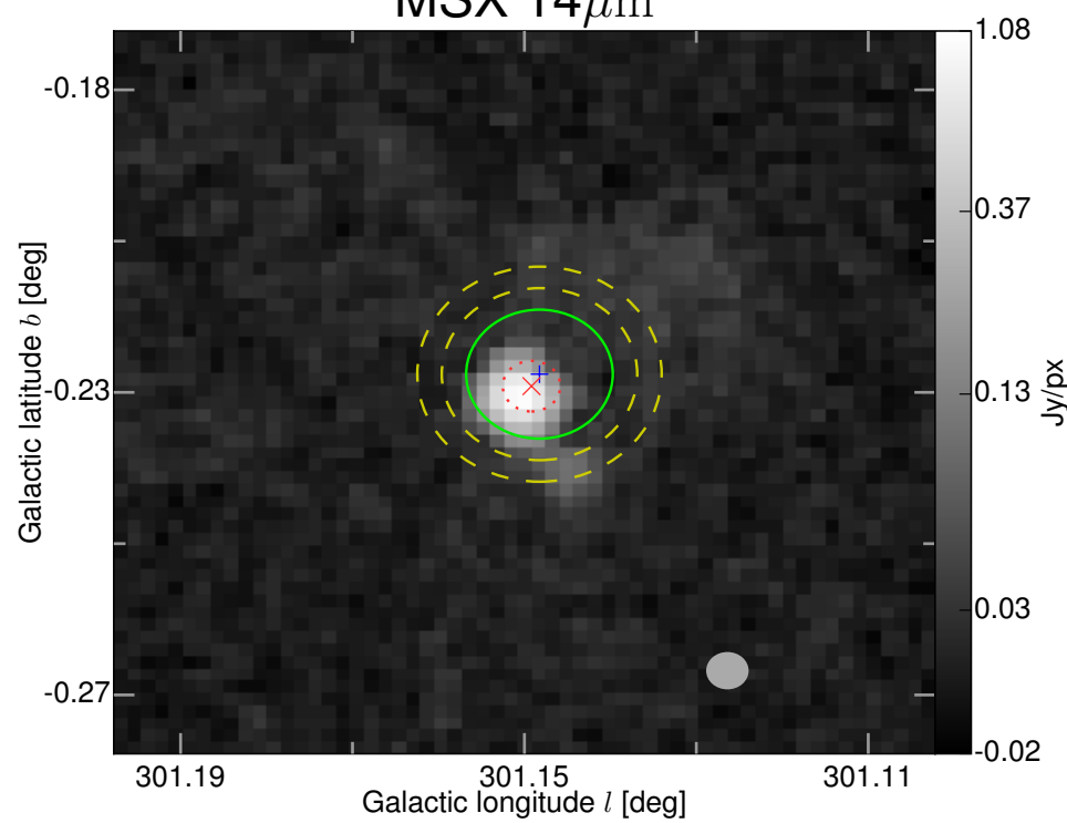
MSX 14\mu\text{m}
