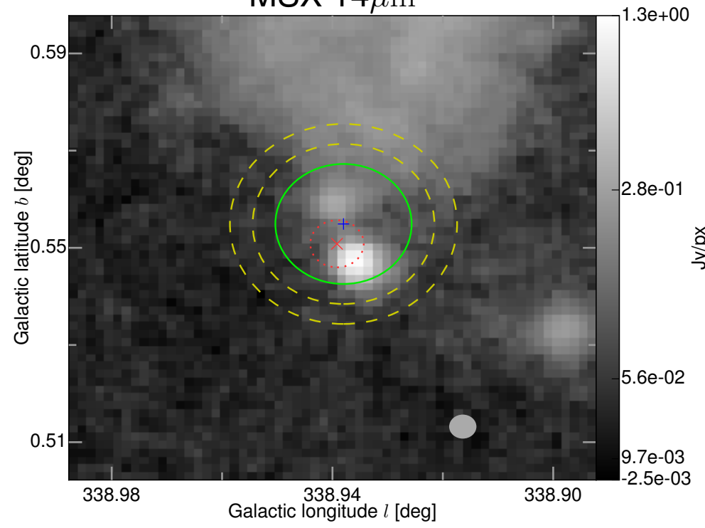
MSX 14\mu\text{m}
