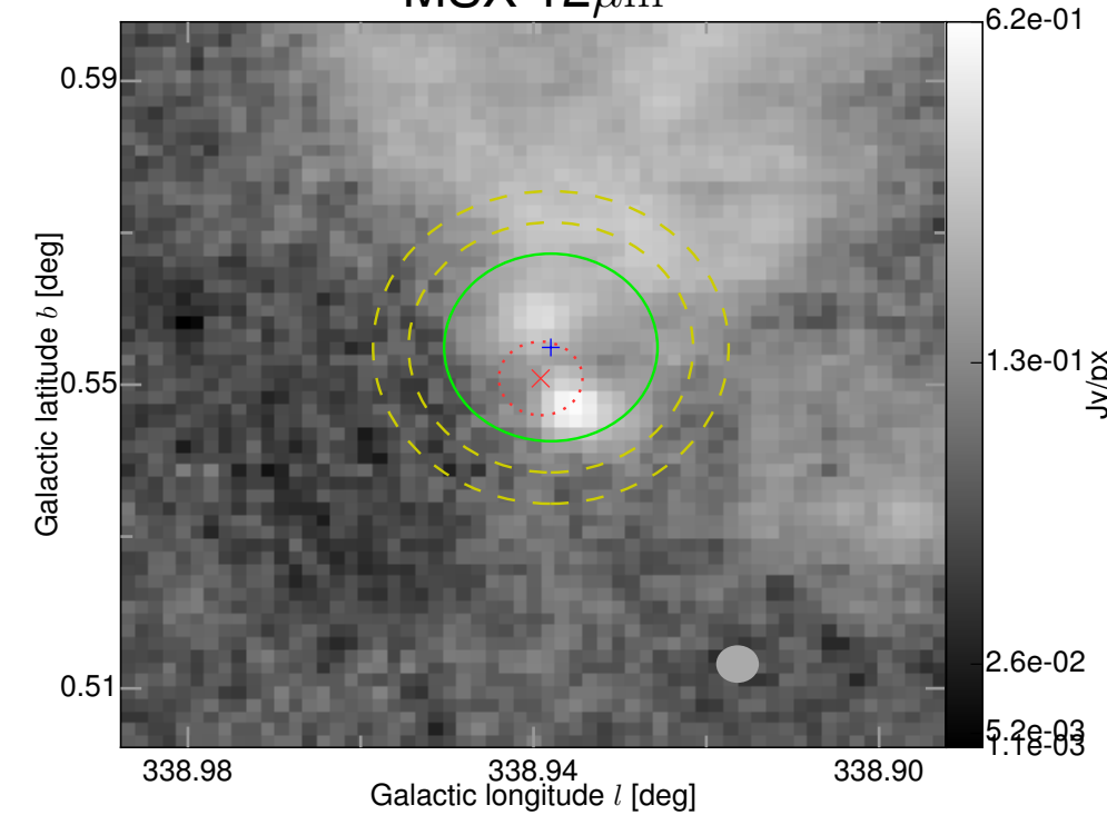
MSX 12\mu\text{m}
