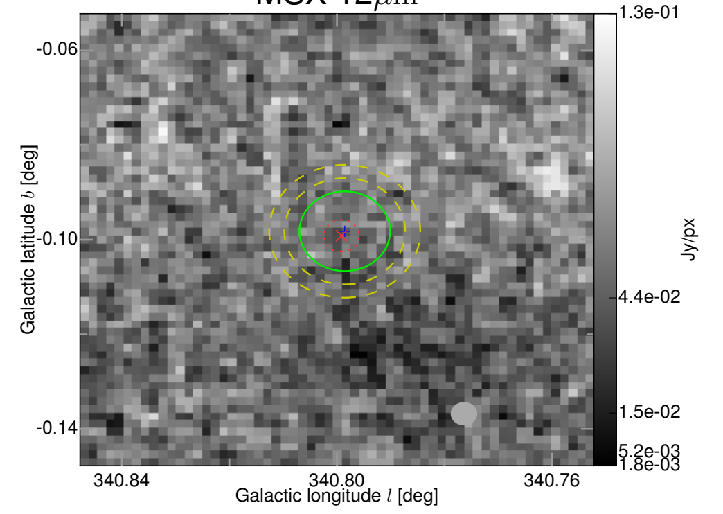
MSX 12\mu\text{m}
