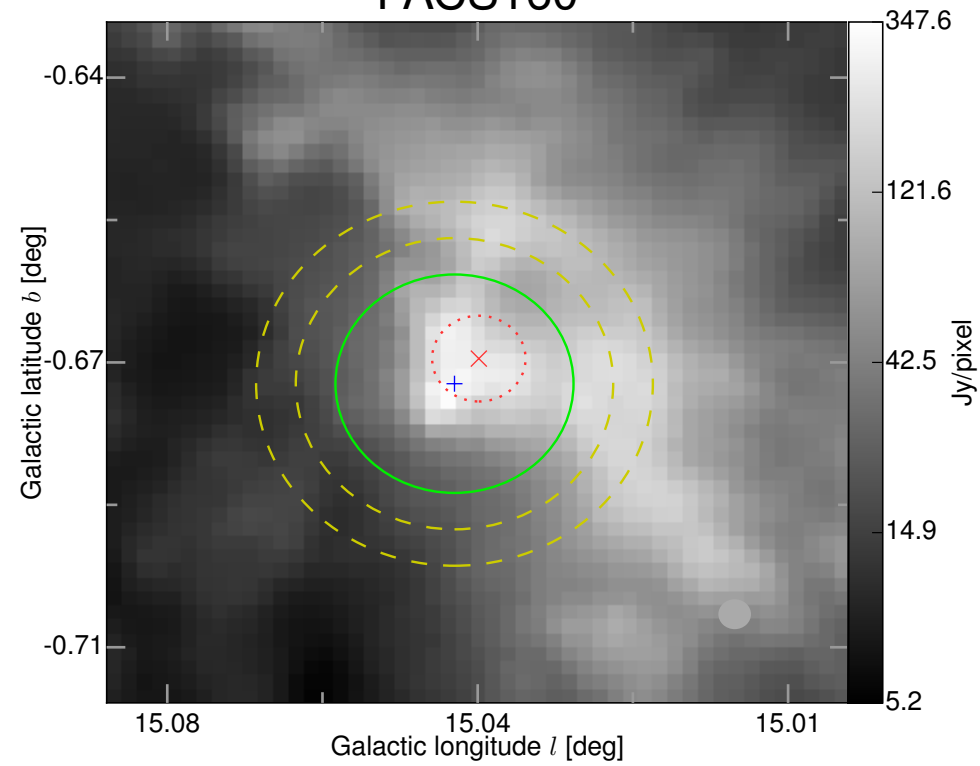
PACS160
