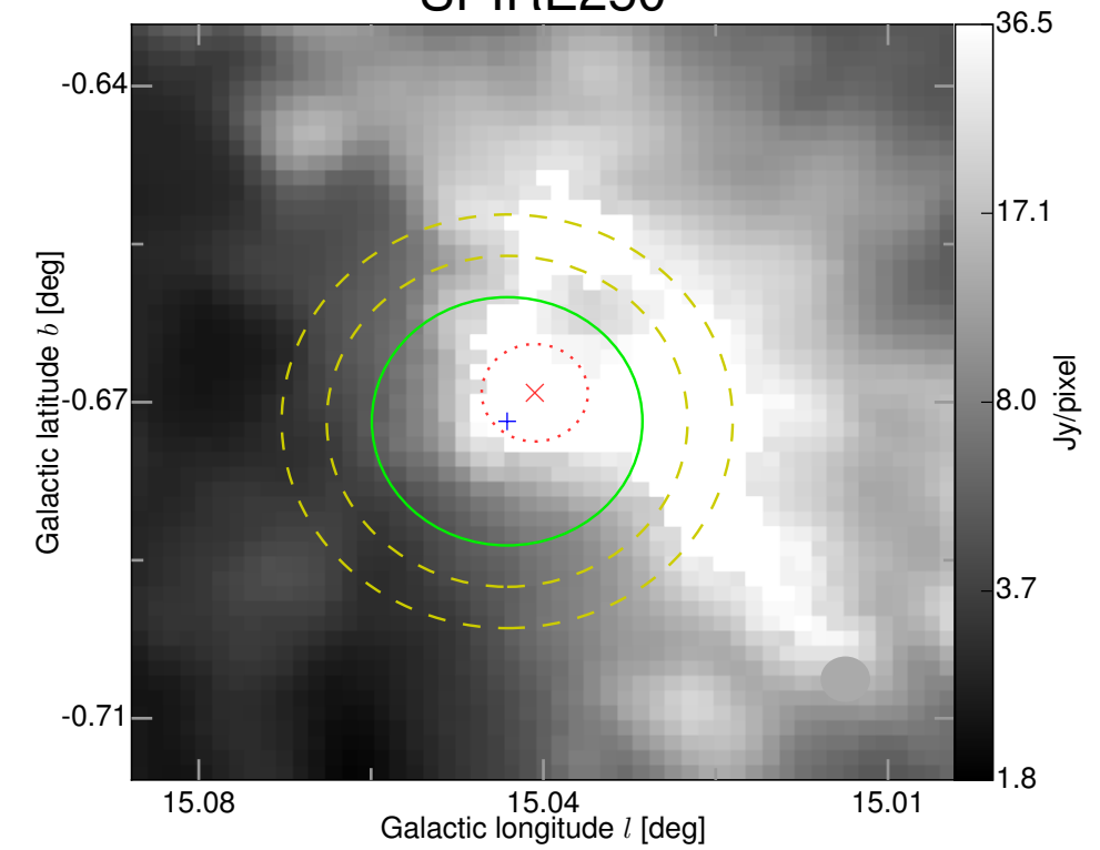
SPIRE250
