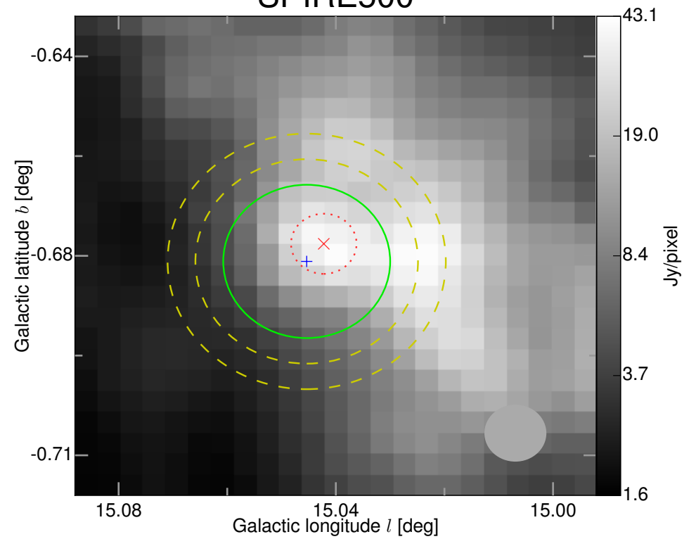
SPIRE500
