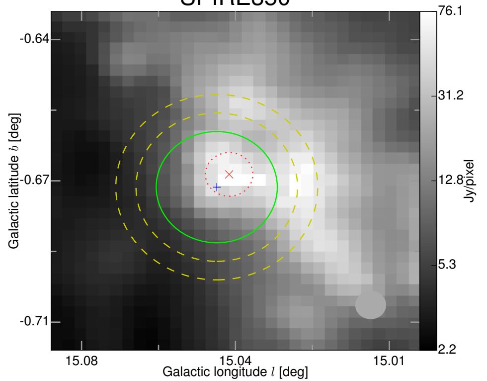
SPIRE350
