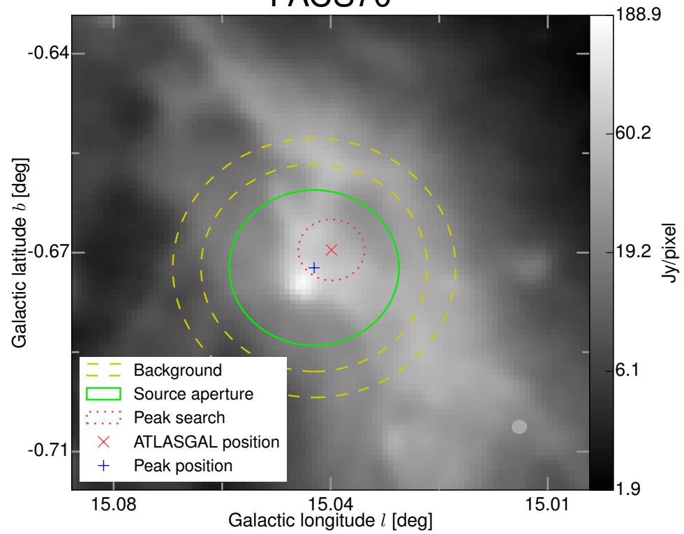
PACS70
