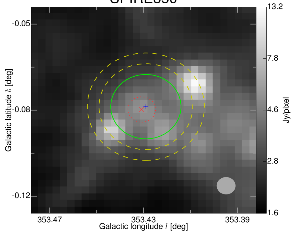
SPIRE350
