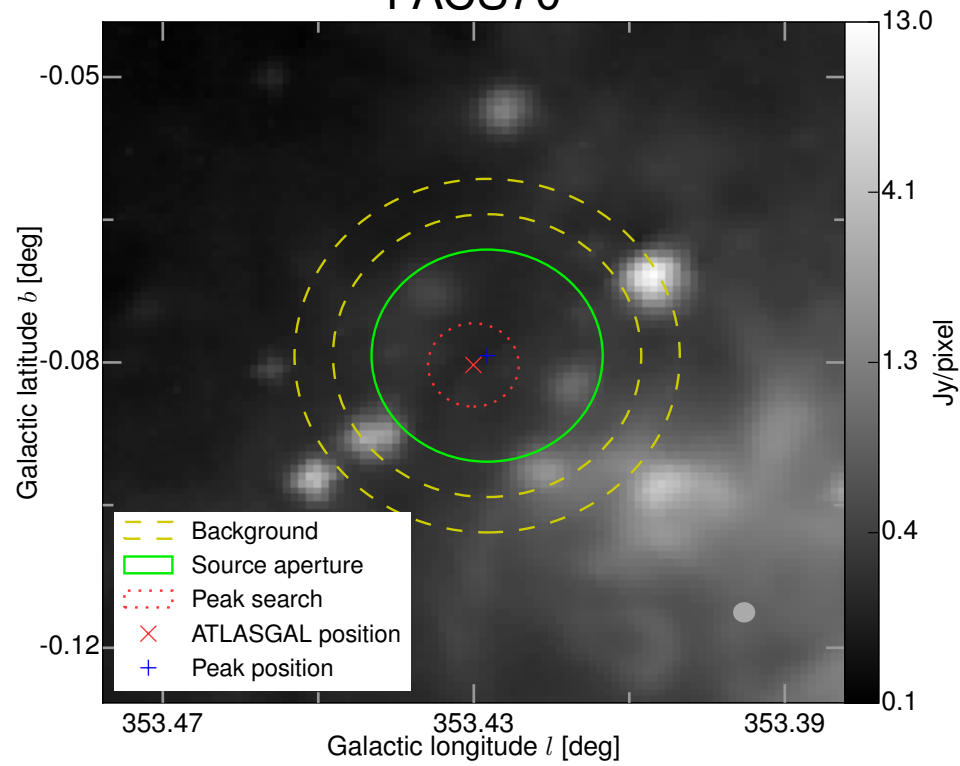
PACS70
