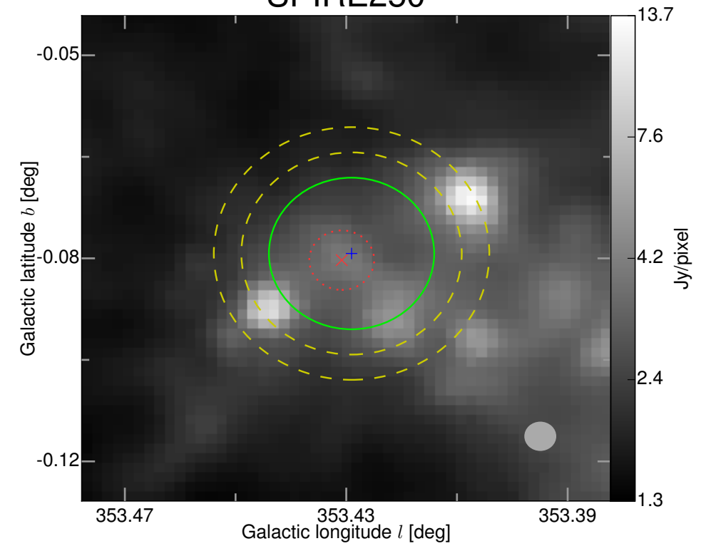
SPIRE250
