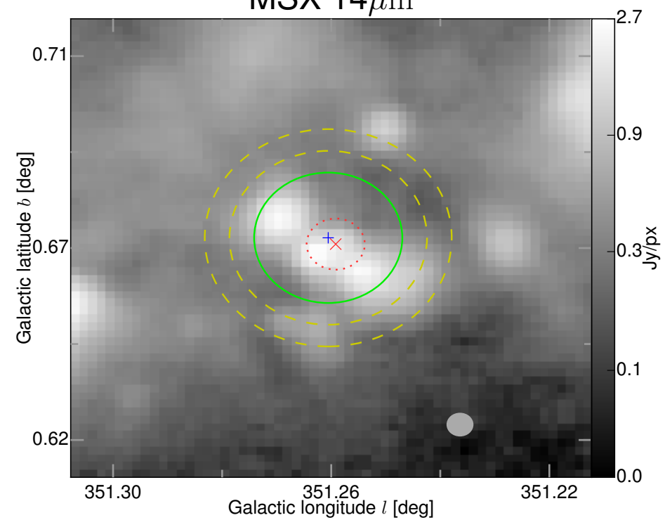
MSX 14 \mu\text{m}
