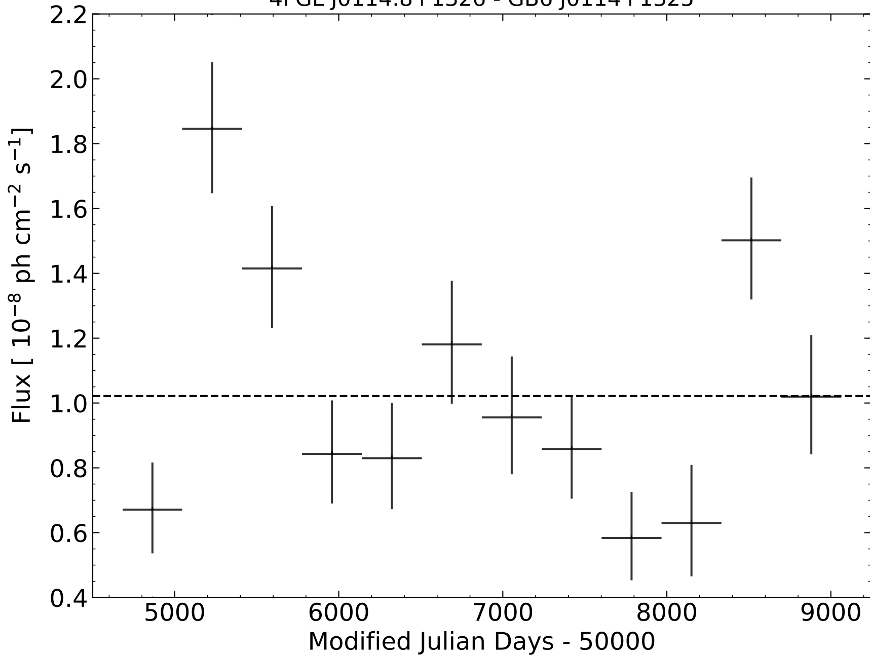
4FGL J0114.8+1326 - GB6 J0114+1325
