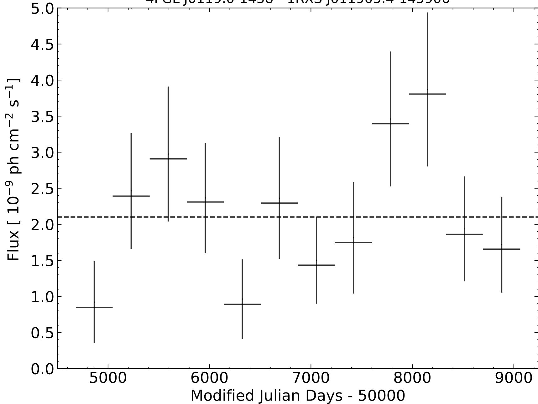
4FGL J0119.0-1458 - 1RXS J011905.4-145906
