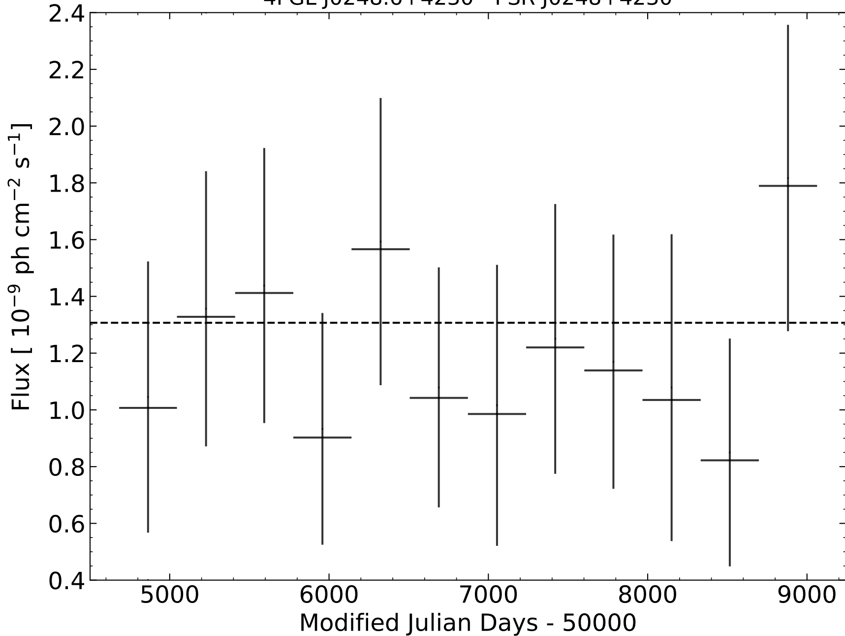
4FGL J0248.6+4230 - PSR J0248+4230
