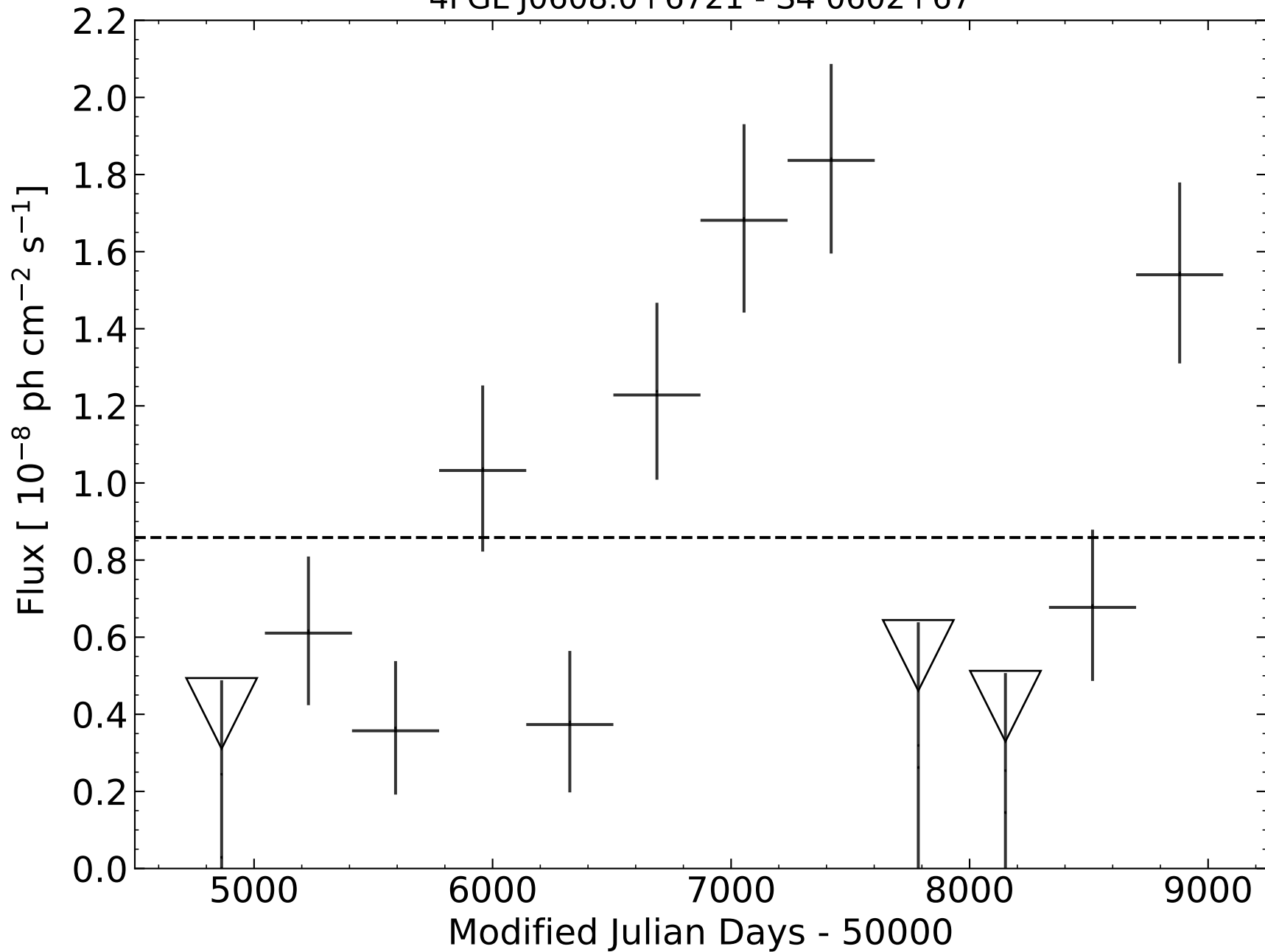
4FGL J0608.0+6721 - S4 0602+67
