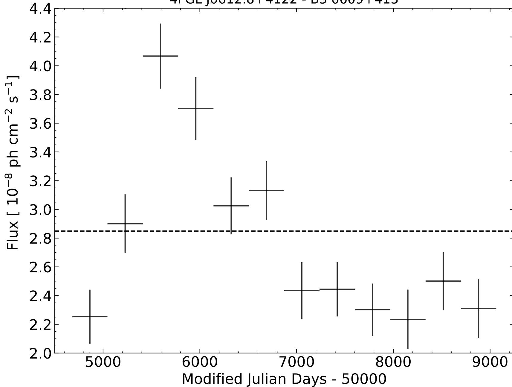
4FGL J0612.8+4122 - B3 0609+413
