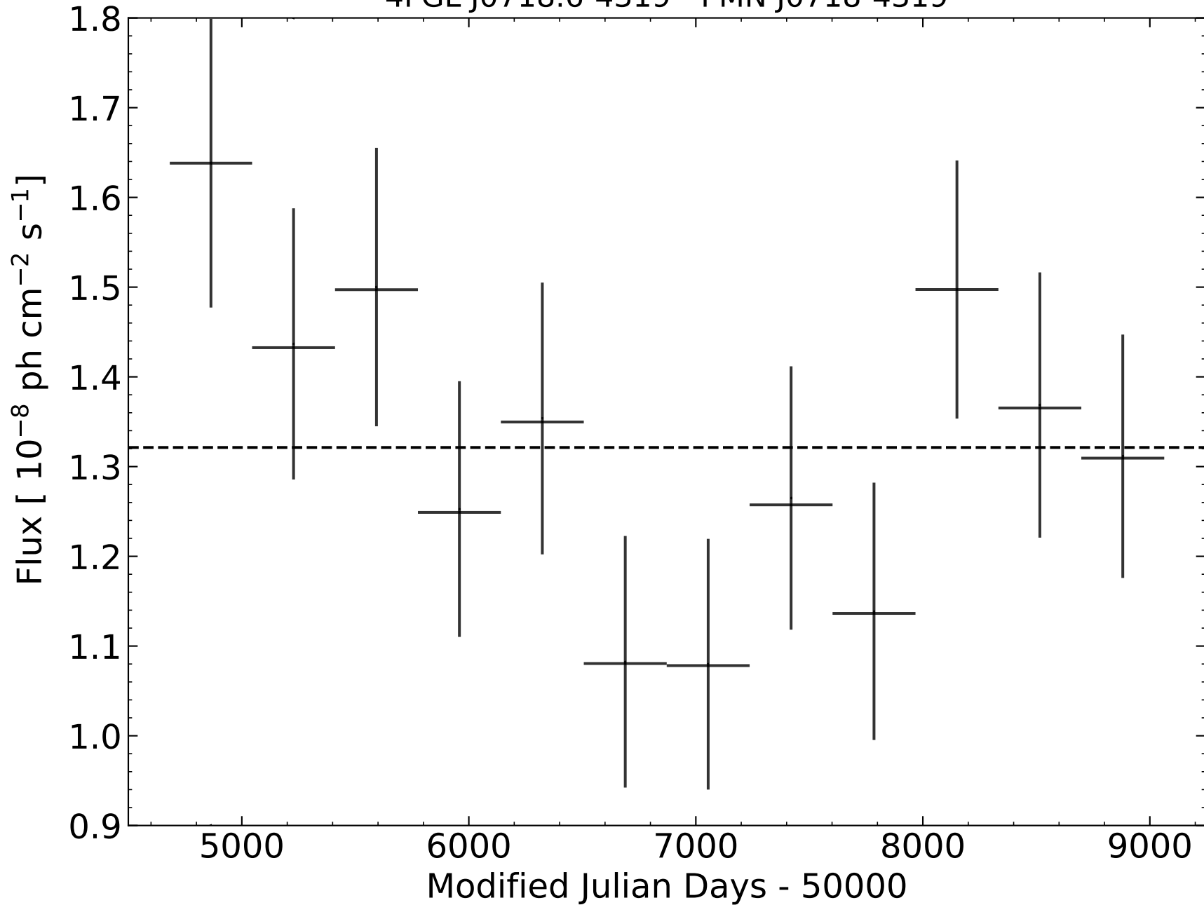
4FGL J0718.6-4319 - PMN J0718-4319
