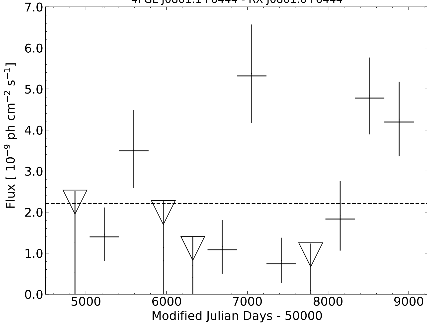
4FGL J0801.1+6444 - RX J0801.0+6444
