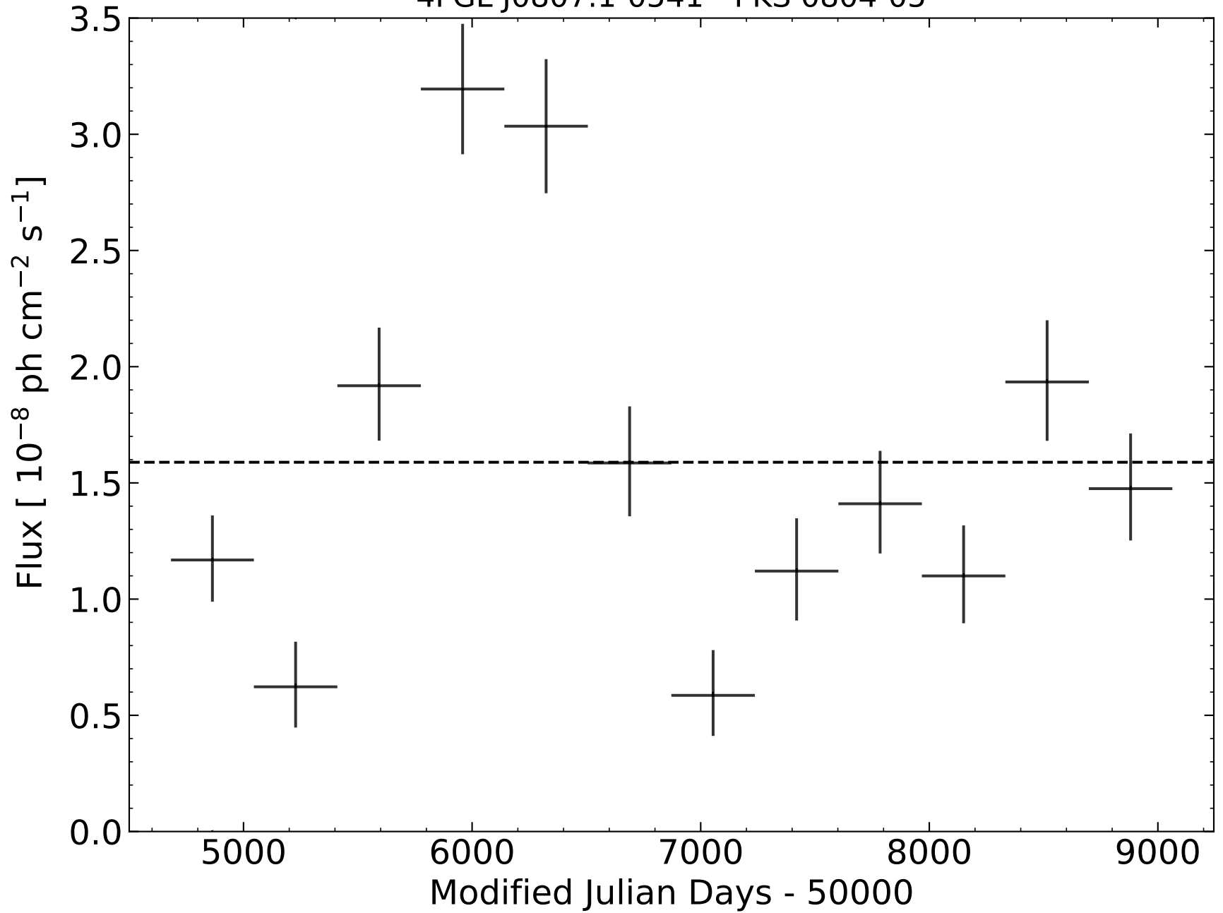
4FGL J0807.1-0541 - PKS 0804-05
