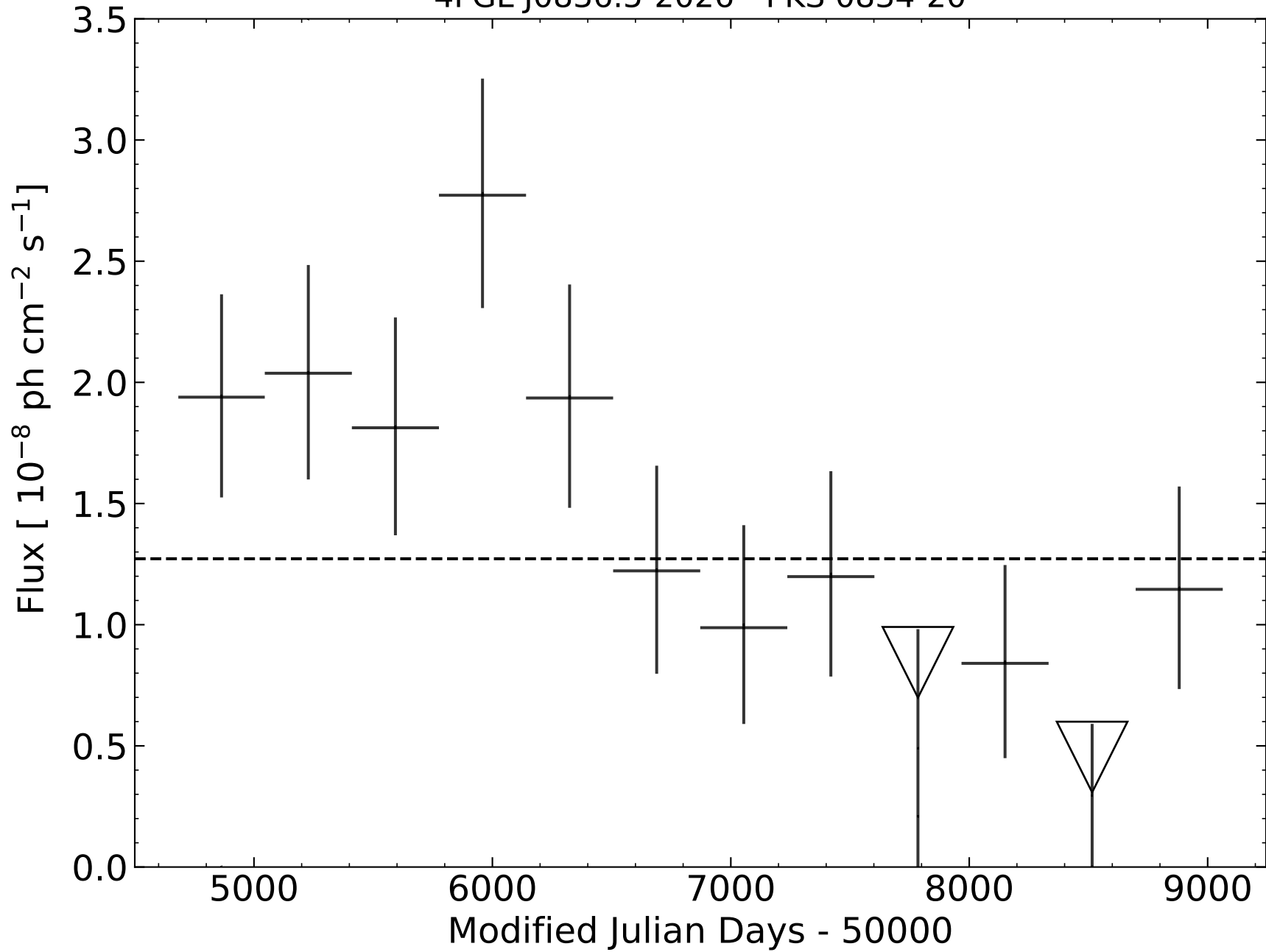
4FGL J0836.5-2026 - PKS 0834-20
