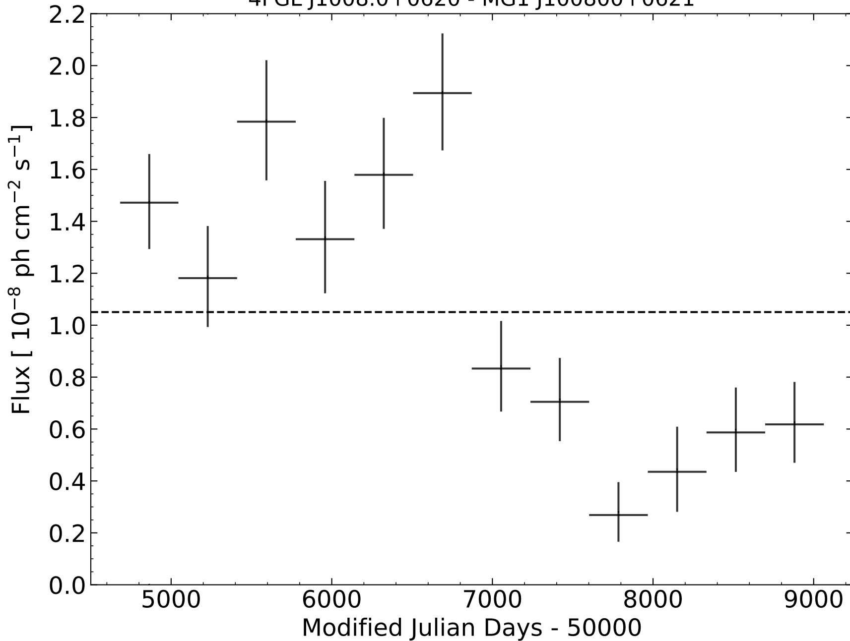
4FGL J1008.0+0620 - MG1 J100800+0621
