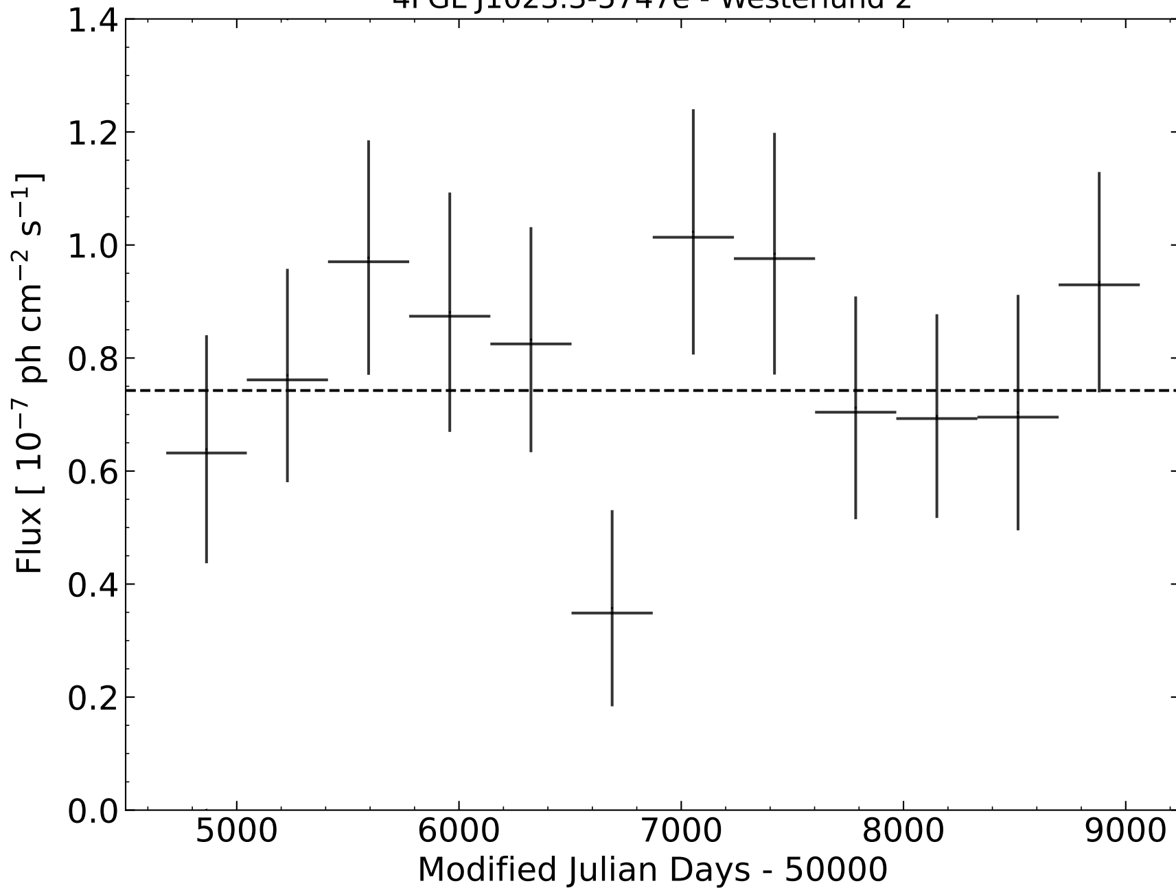
4FGL J1023.3-5747e - Westerlund 2
