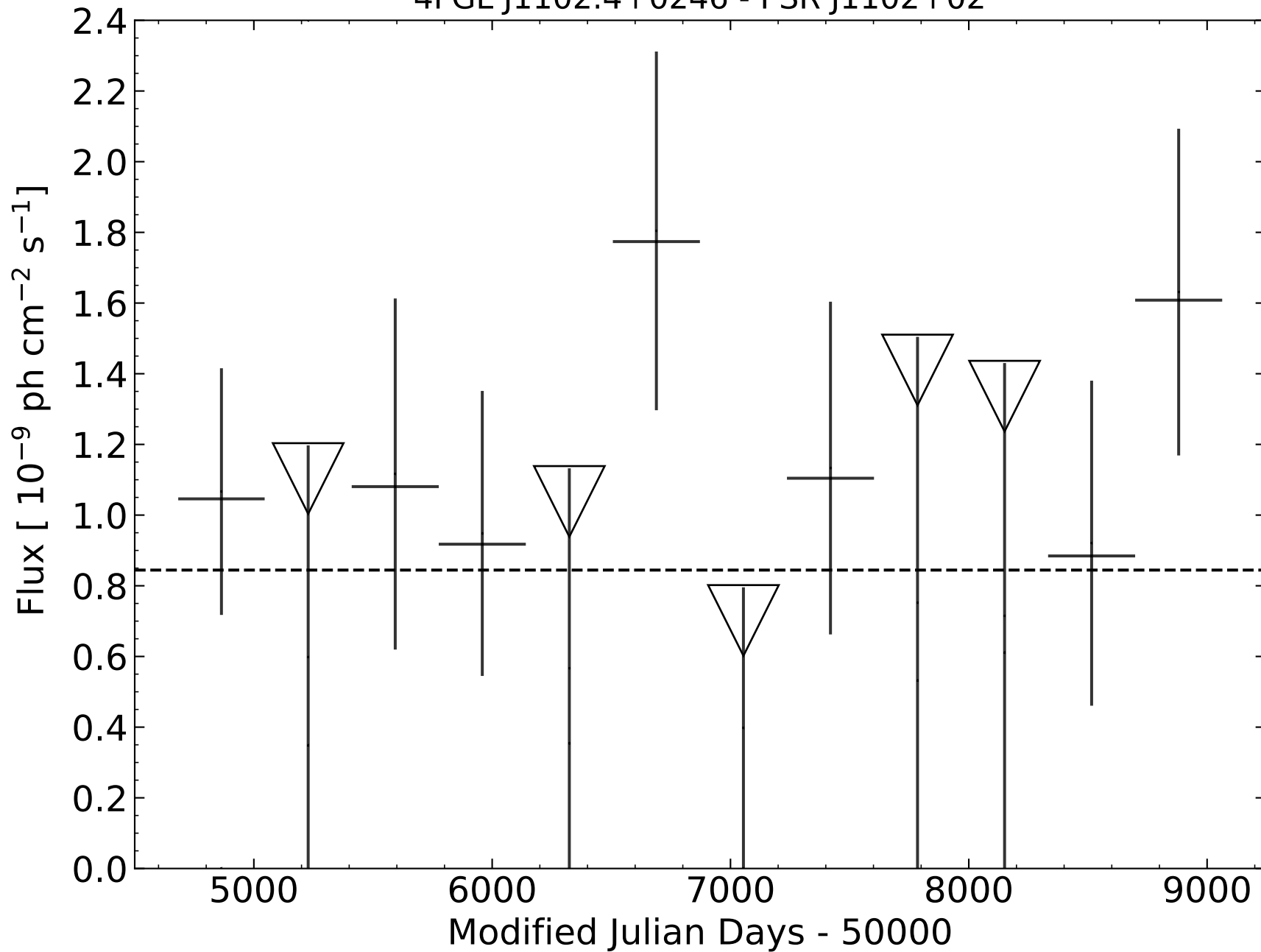
4FGL J1102.4+0246 - PSR J1102+02
