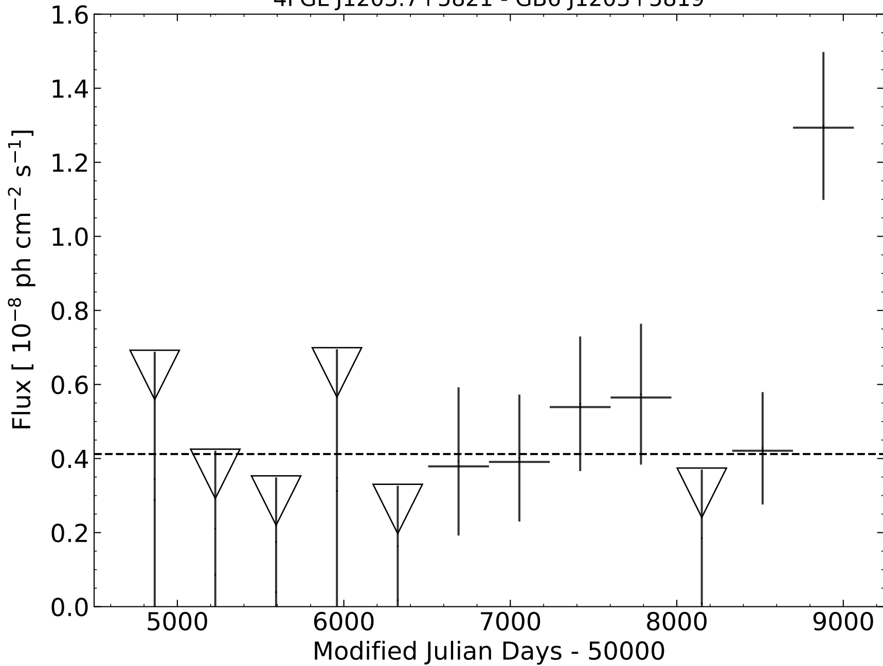
4FGL J1203.7+5821 - GB6 J1203+5819
