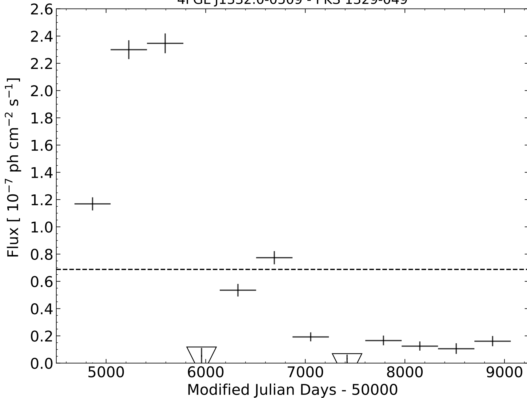
4FGL J1332.0-0509 - PKS 1329-049
