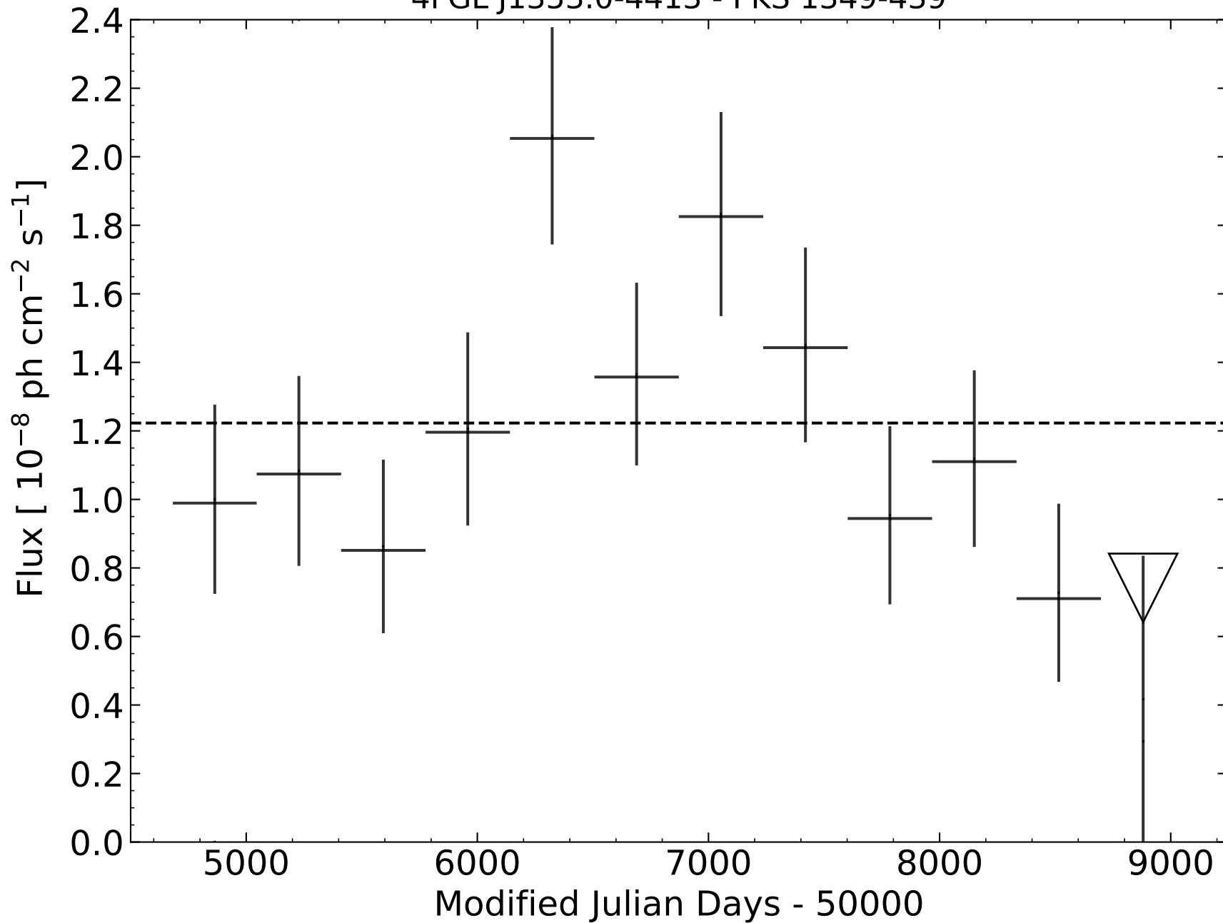
4FGL J1353.0-4413 - PKS 1349-439
