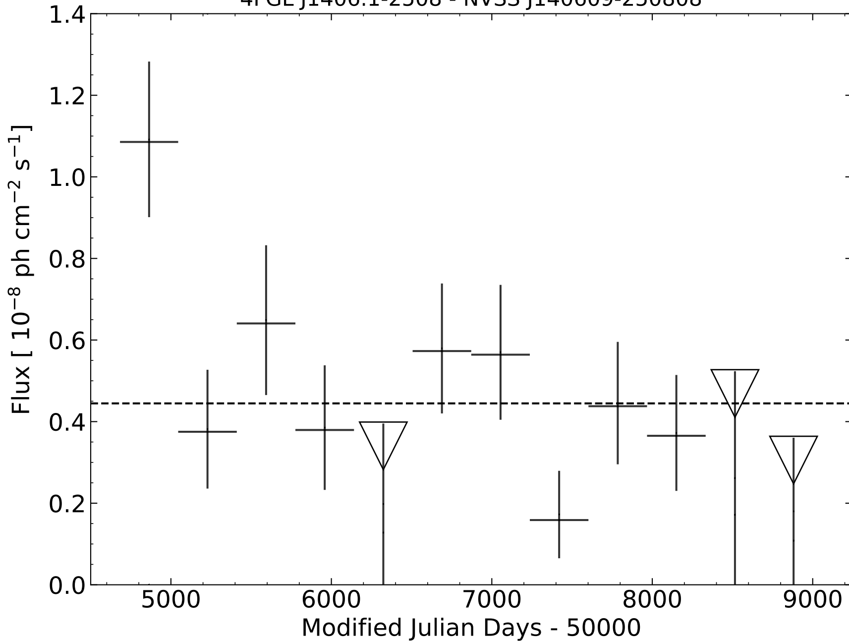
4FGL J1406.1-2508 - NVSS J140609-250808
