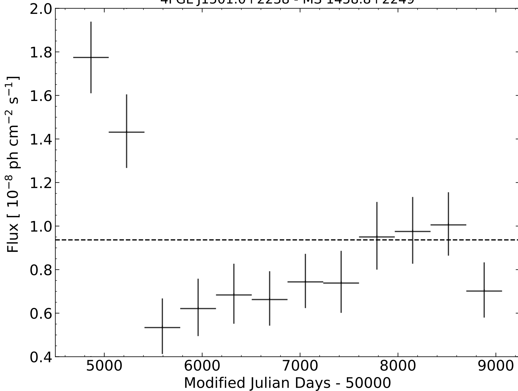
4FGL J1501.0+2238 - MS 1458.8+2249
