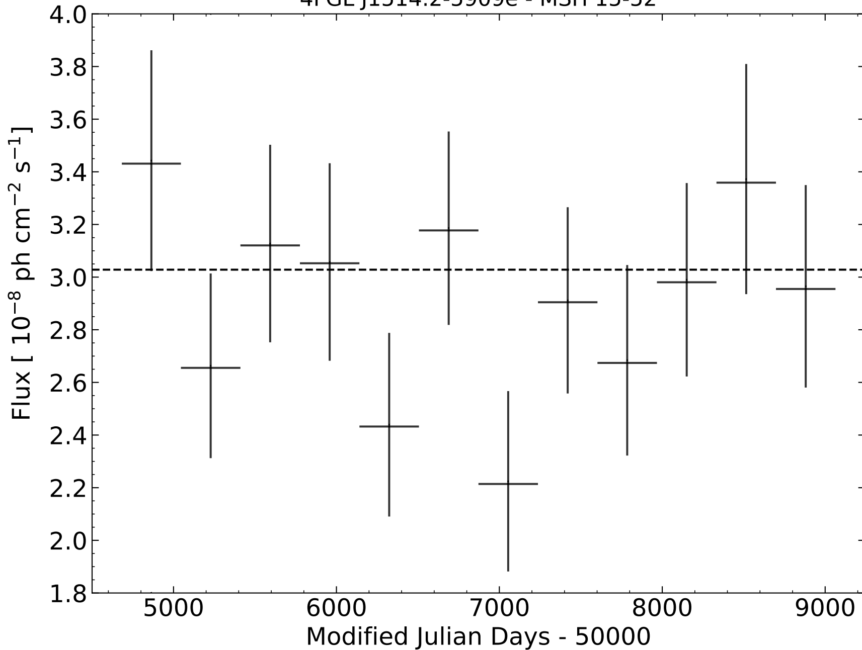
4FGL J1514.2-5909e - MSH 15-52
