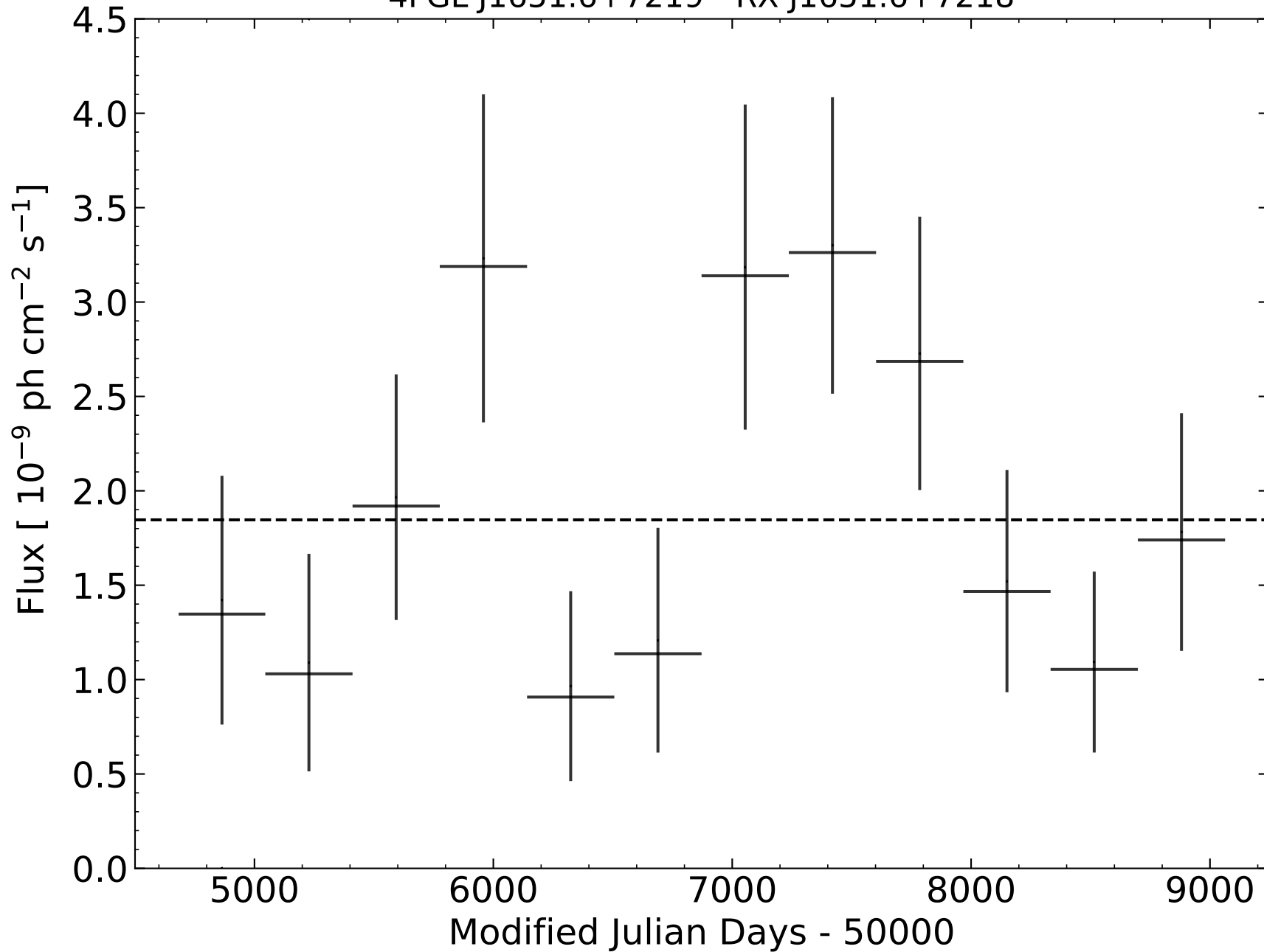
4FGL J1651.6+7219 - RX J1651.6+7218
