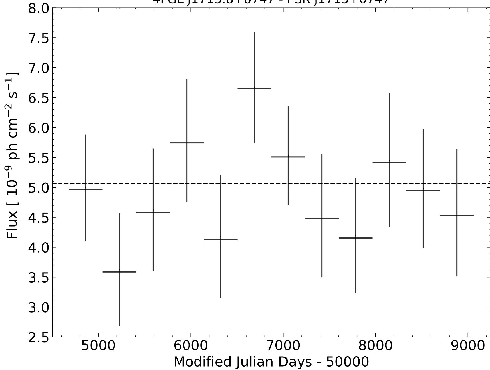
4FGL J1713.8+0747 - PSR J1713+0747
