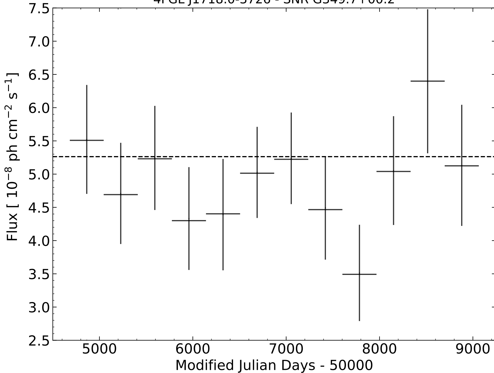
4FGL J1718.0-3726 - SNR G349.7+00.2
