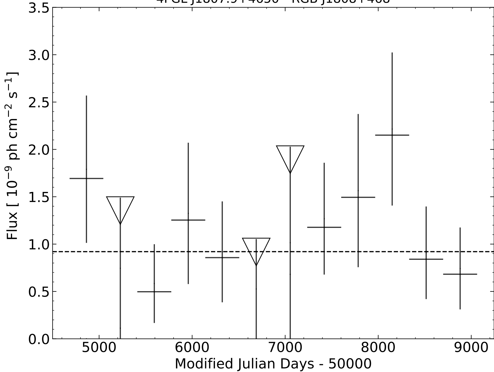
4FGL J1807.9+4650 - RGB J1808+468
