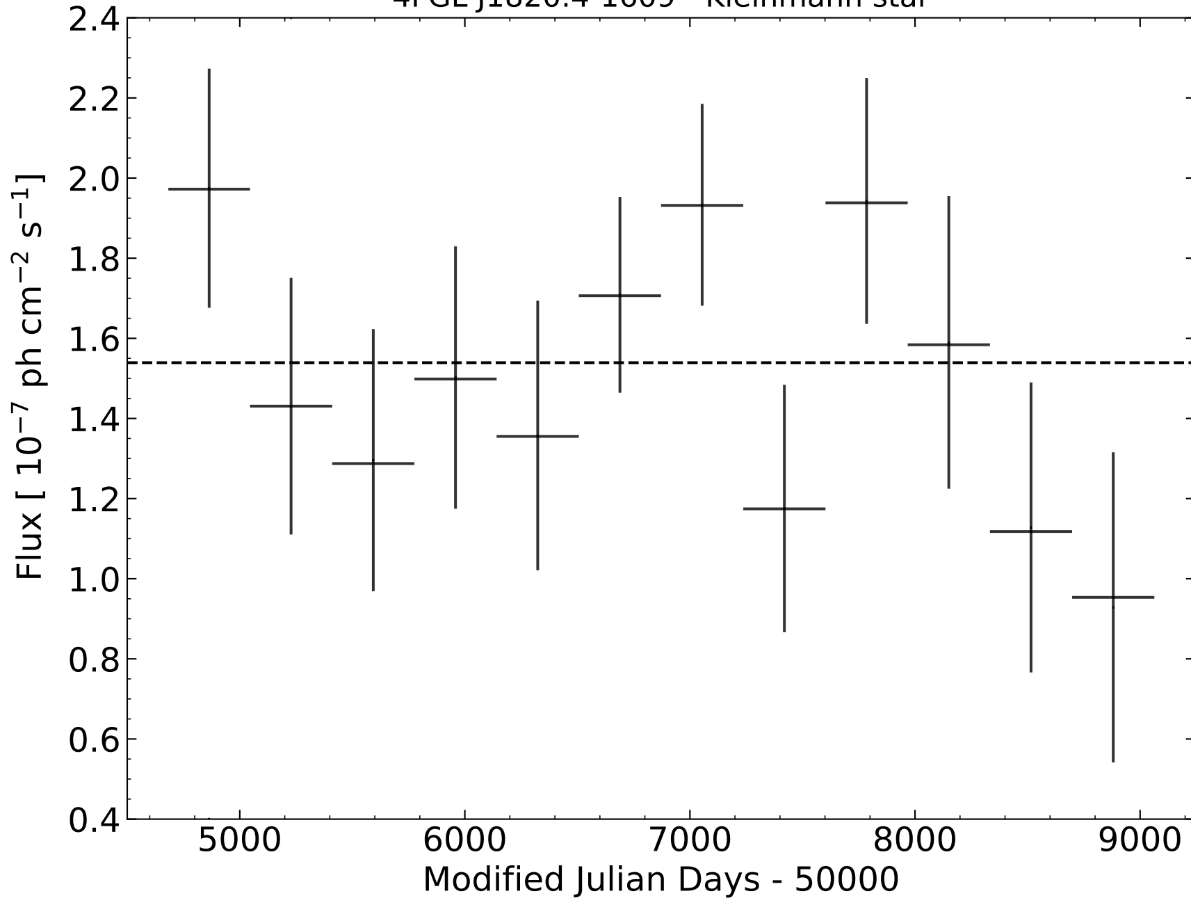
4FGL J1820.4-1609 - Kleinmann star
