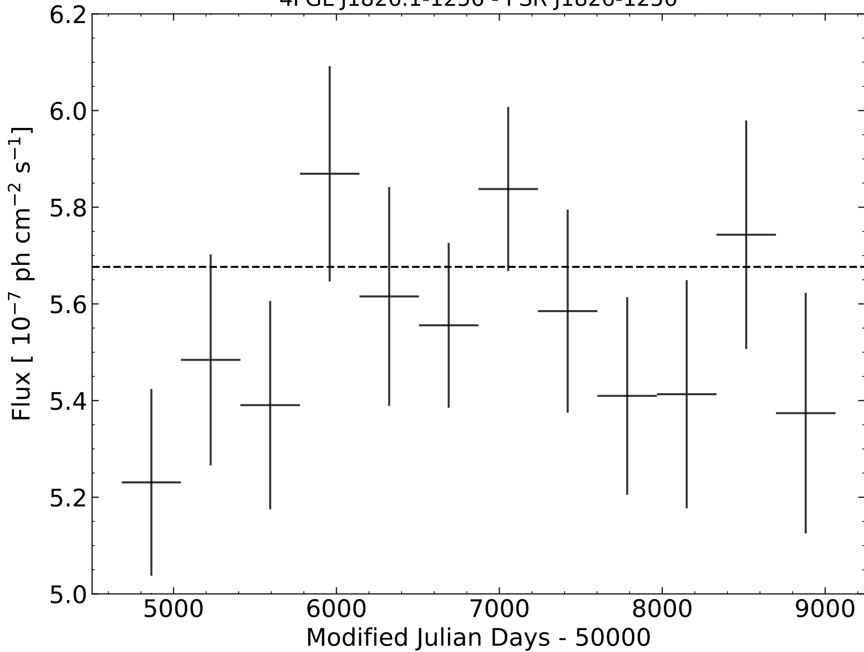
4FGL J1826.1-1256 - PSR J1826-1256
