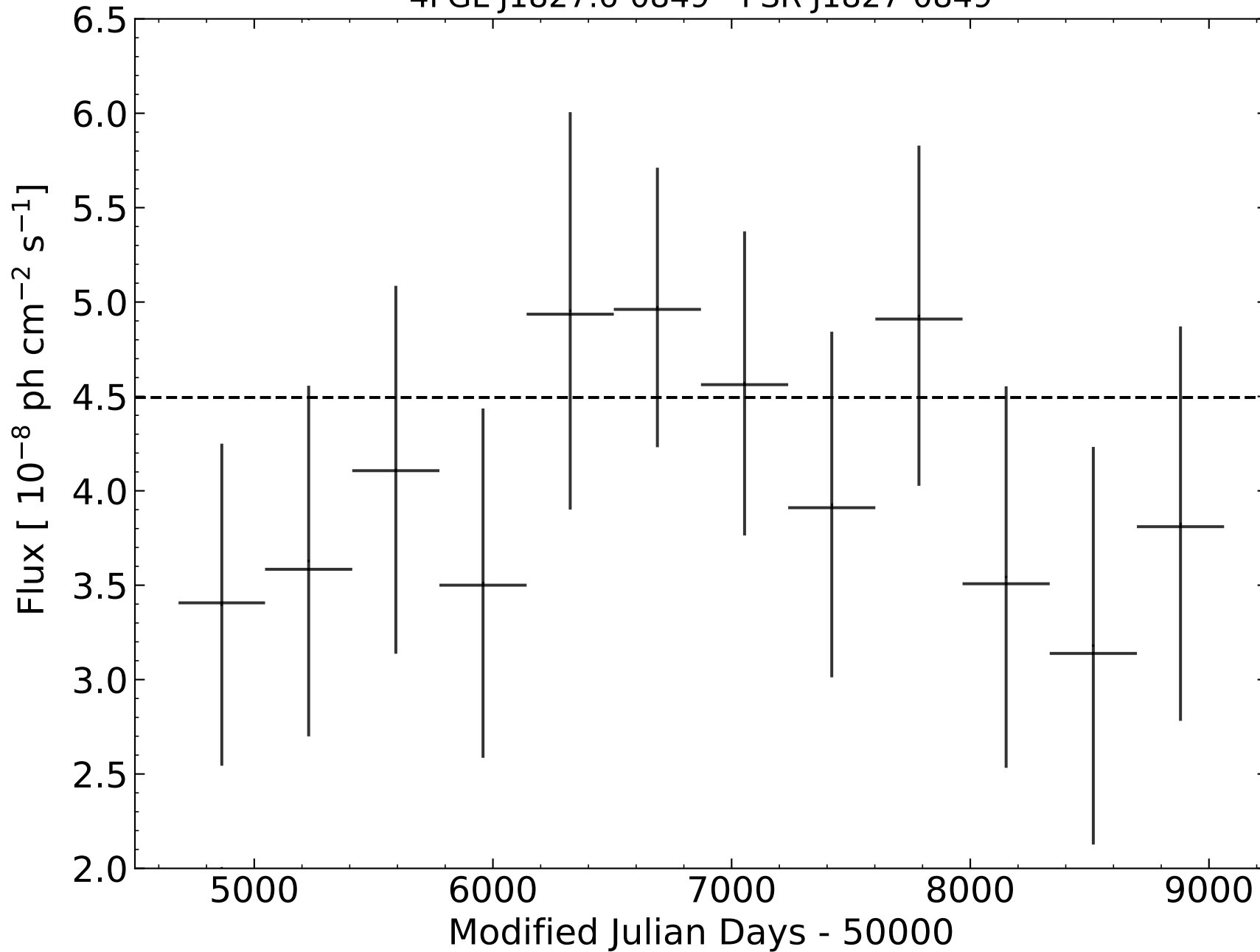
4FGL J1827.6-0849 - PSR J1827-0849
