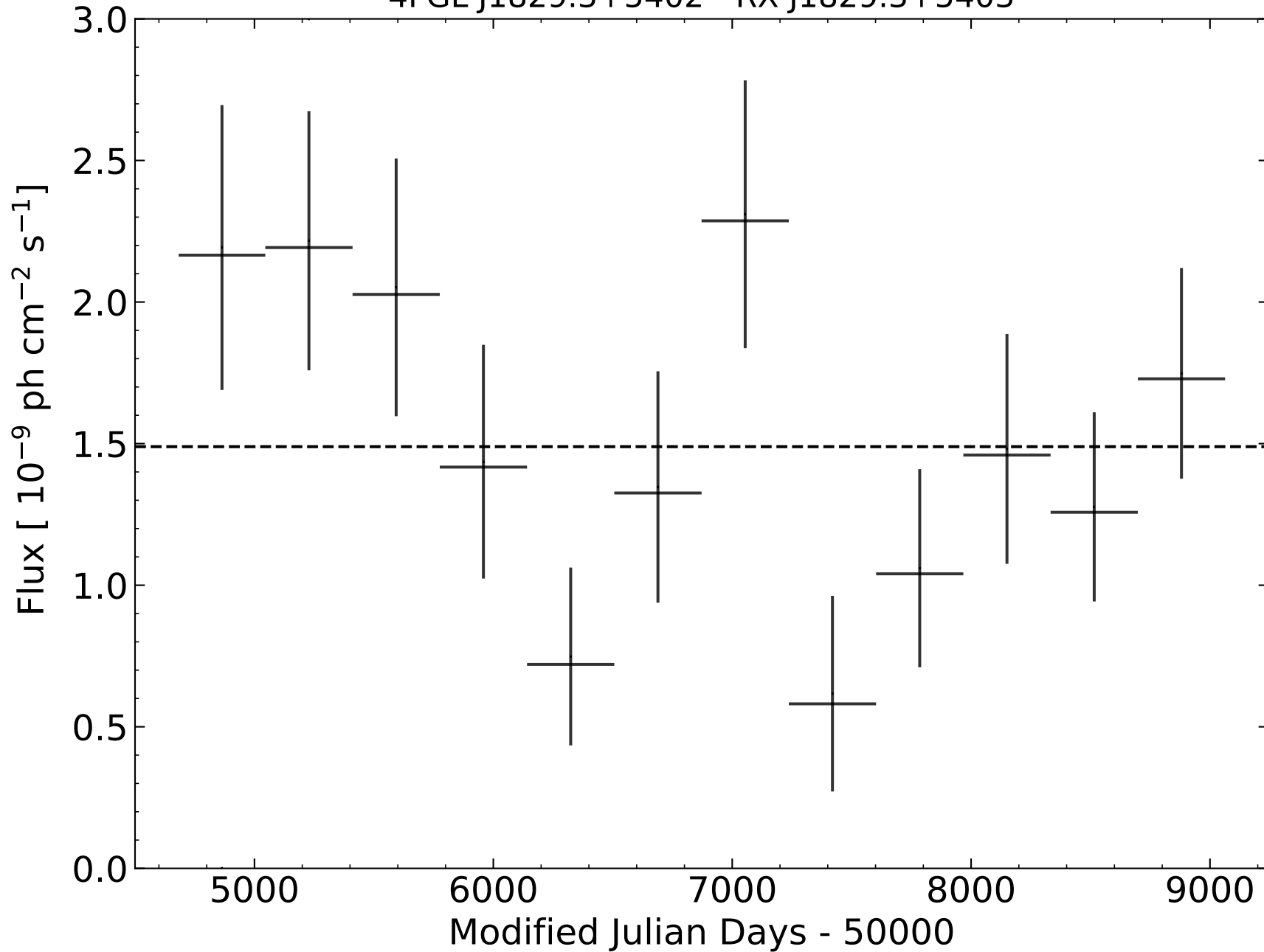
4FGL J1829.3+5402 - RX J1829.3+5403
