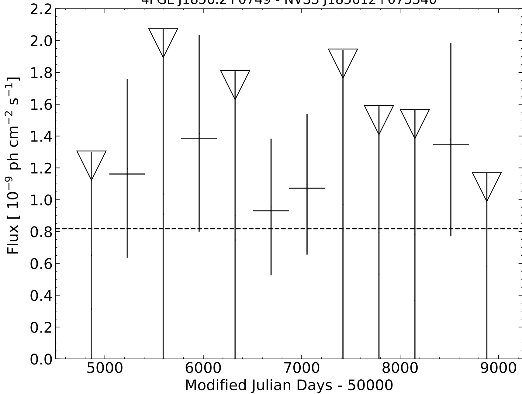
4FGL J1856.2+0749 - NVSS J185612+075340
