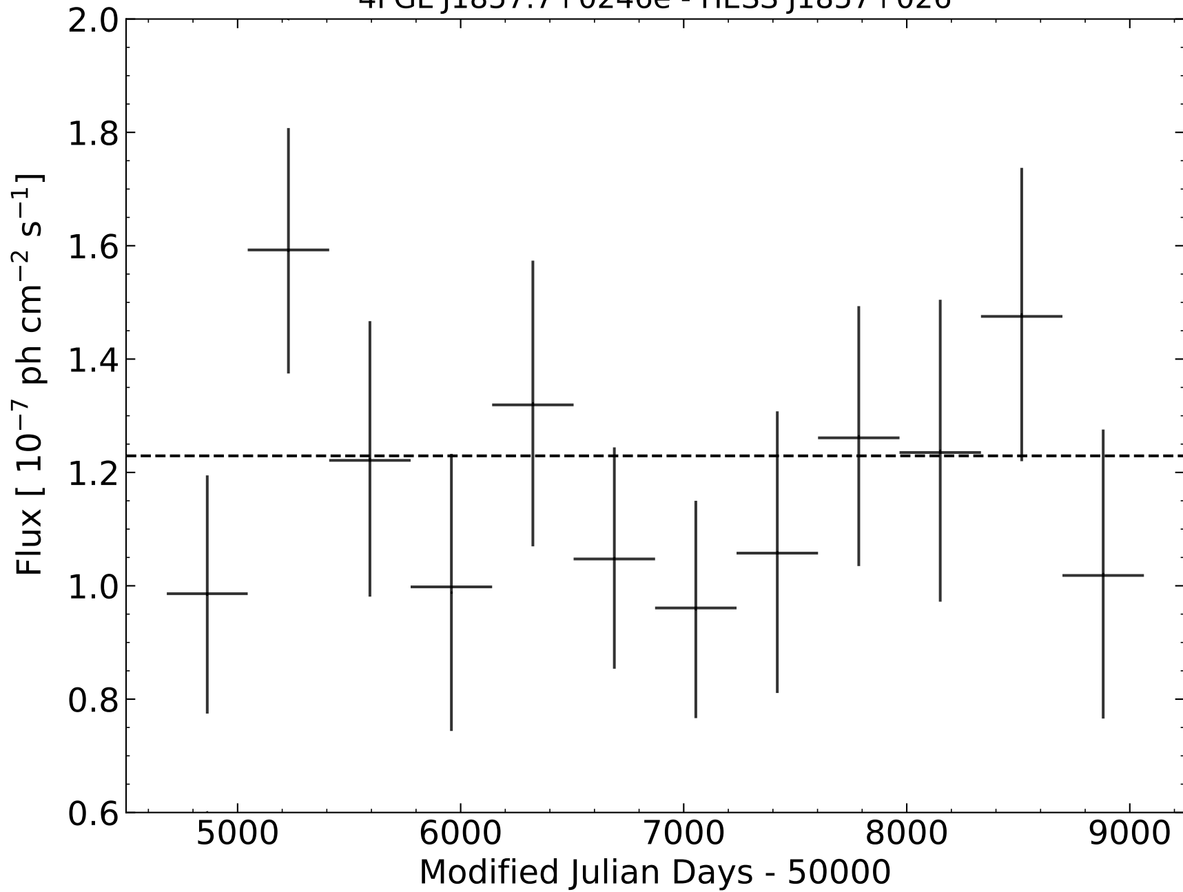
4FGL J1857.7+0246e - HESS J1857+026
