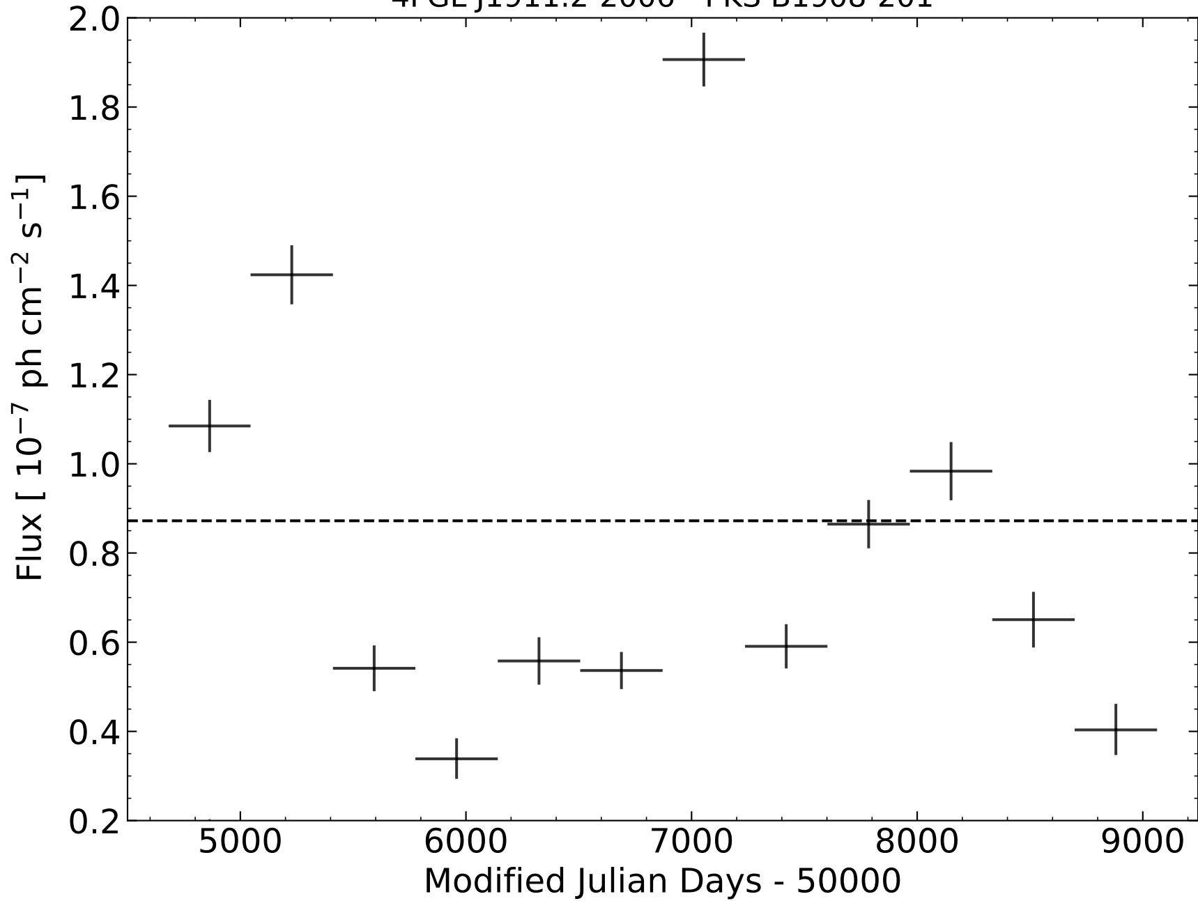
4FGL J1911.2-2006 - PKS B1908-201
