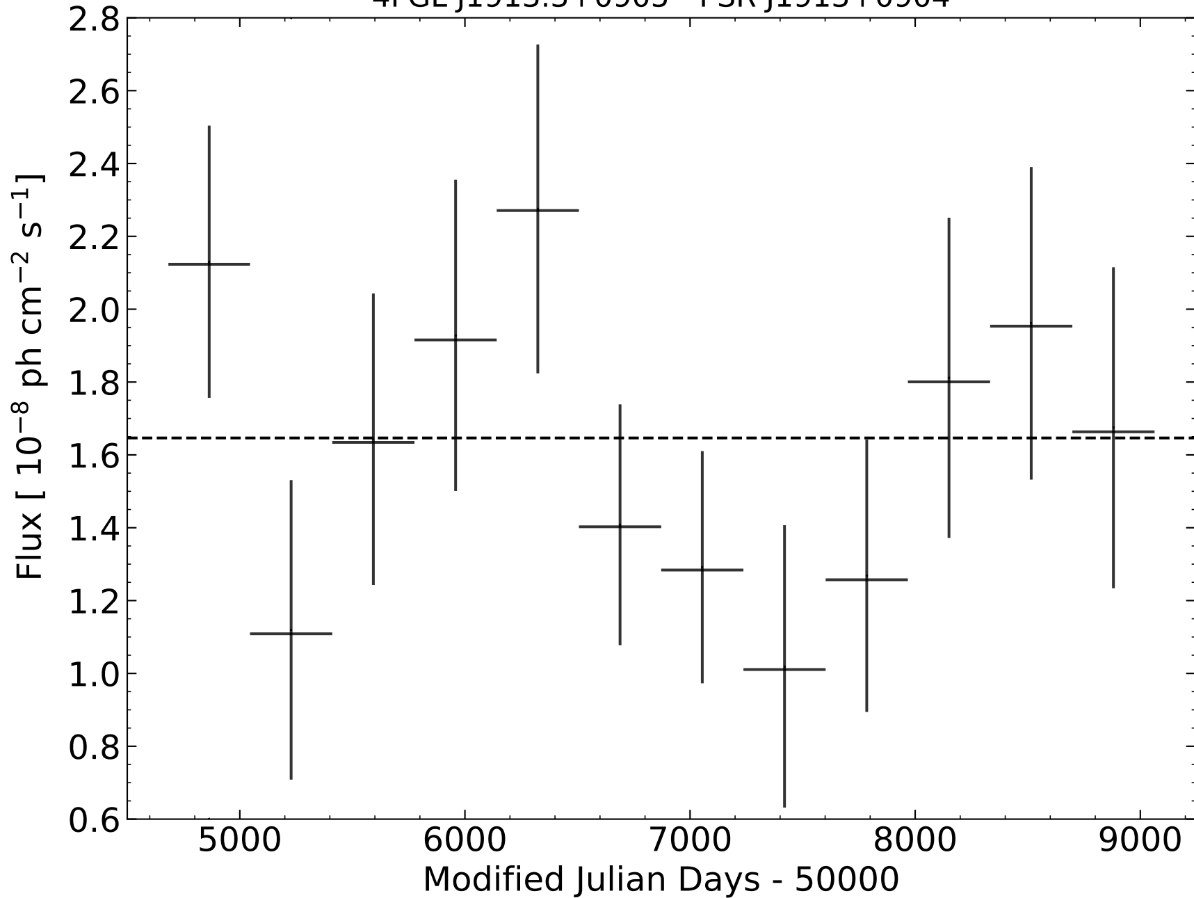
4FGL J1913.3+0905 - PSR J1913+0904
