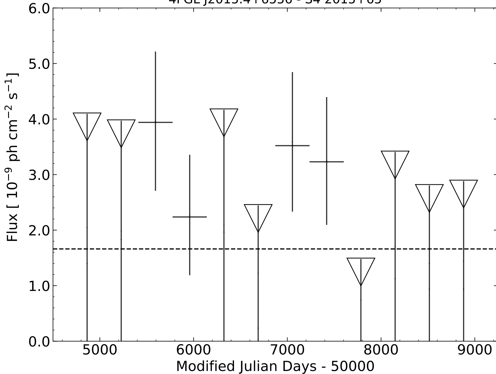
4FGL J2015.4+6556 - S4 2015+65
