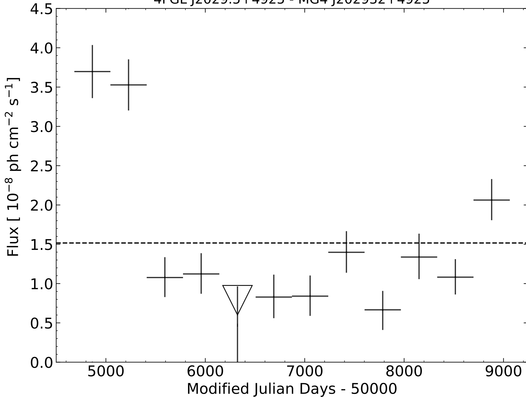
4FGL J2029.5+4925 - MG4 J202932+4925
