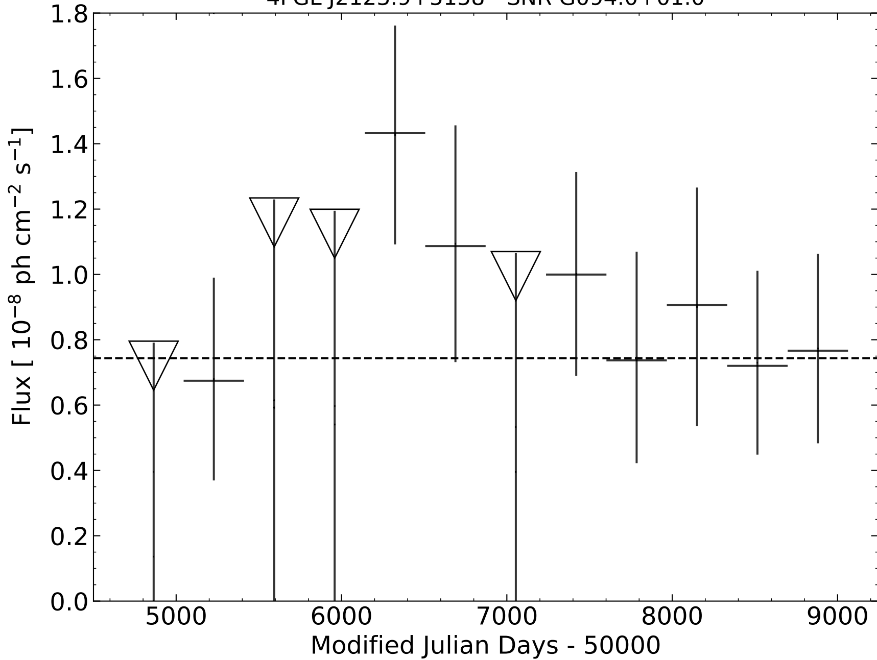
4FGL J2123.9+5158 - SNR G094.0+01.0
