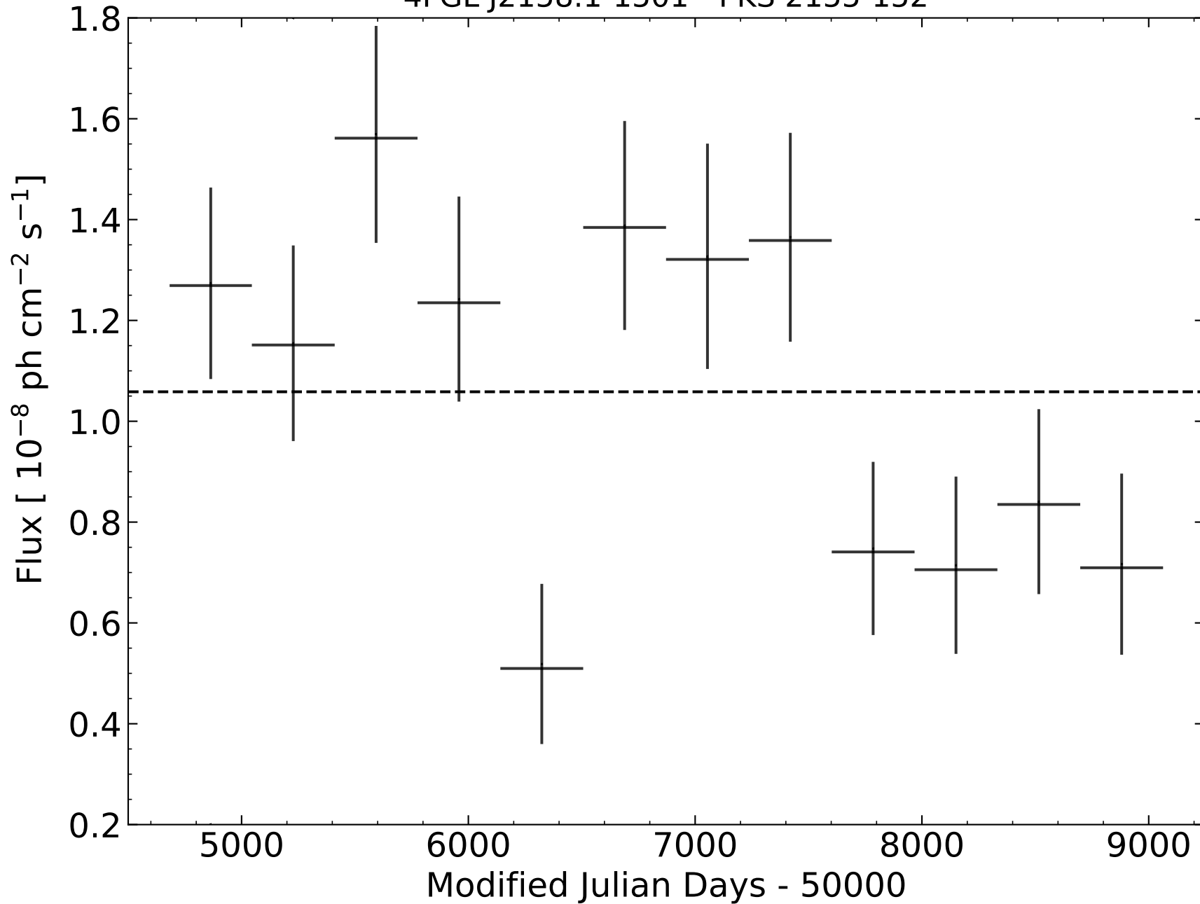
4FGL J2158.1-1501 - PKS 2155-152
